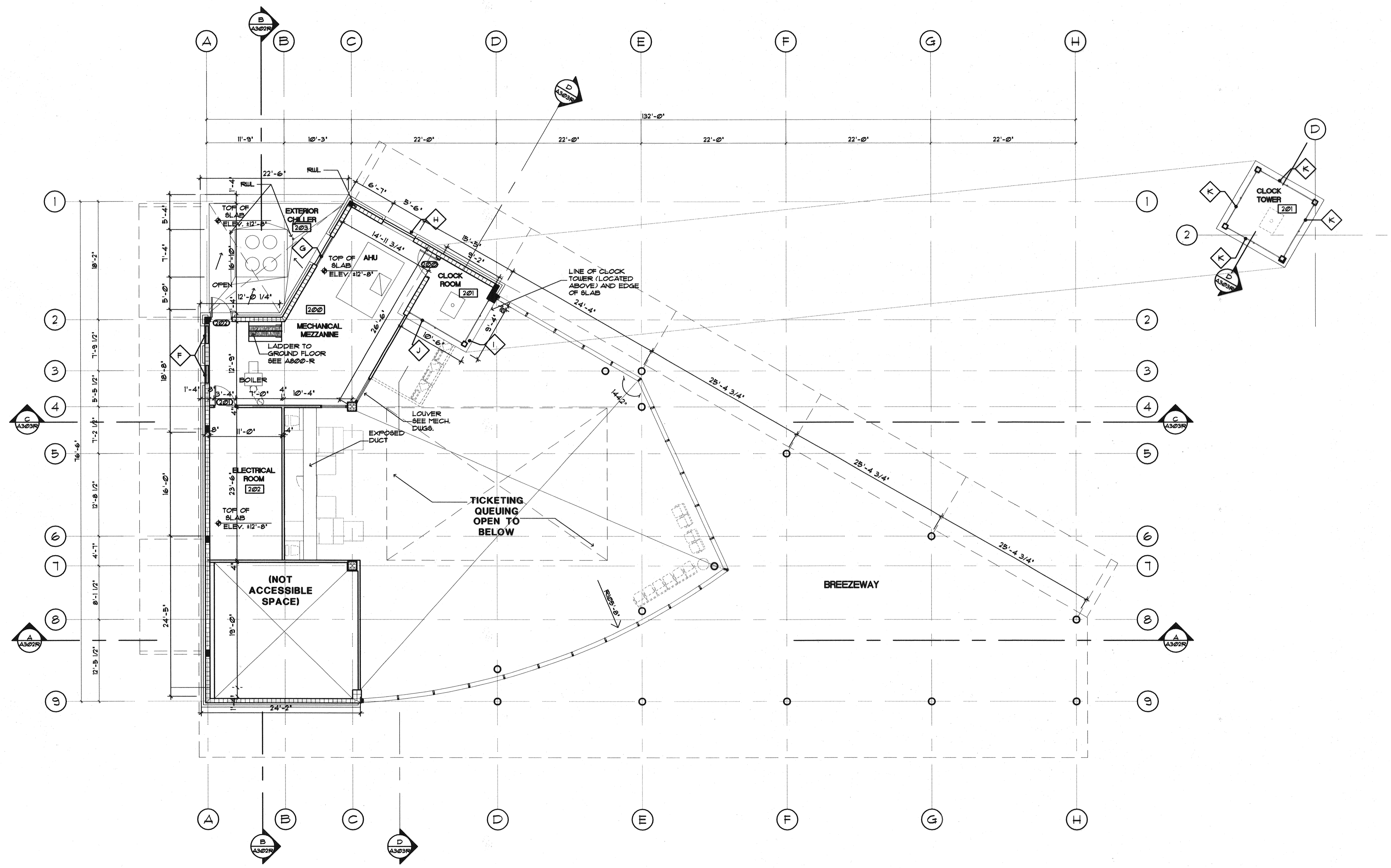
MEZZANINE FLOOR PLAN SCALE: 1/8" = 1'-0"
