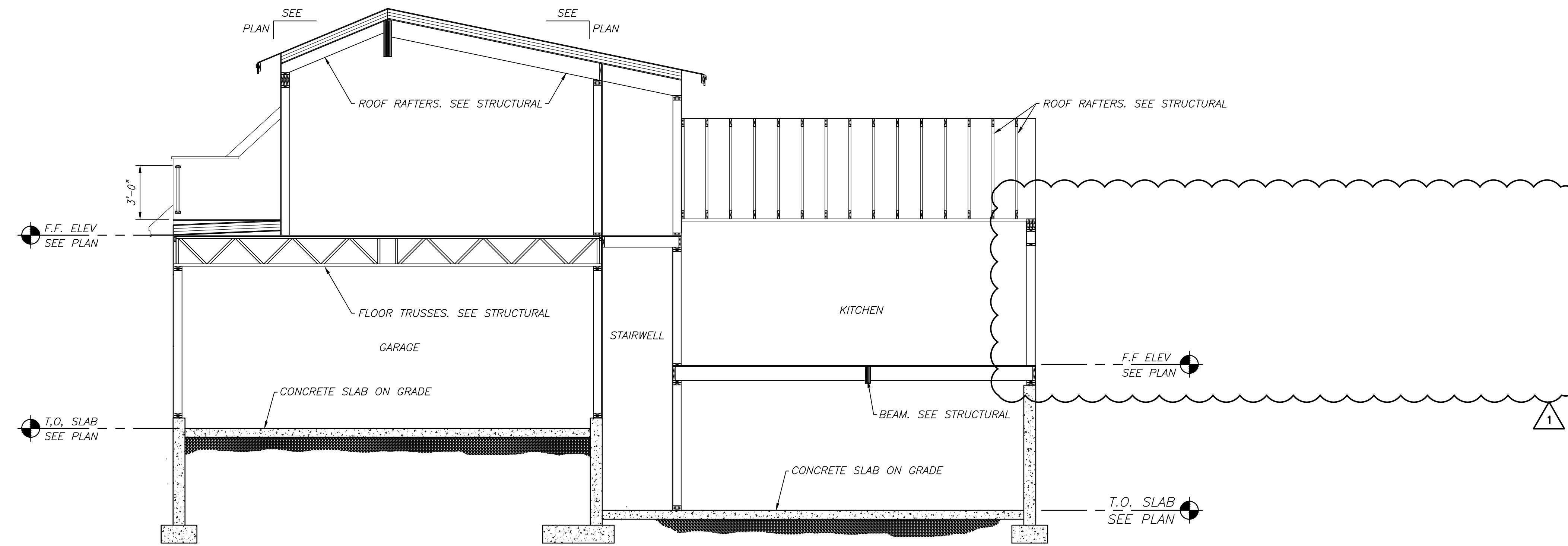
A2 SECTION SCALE: 1/4" = 1'-0"
