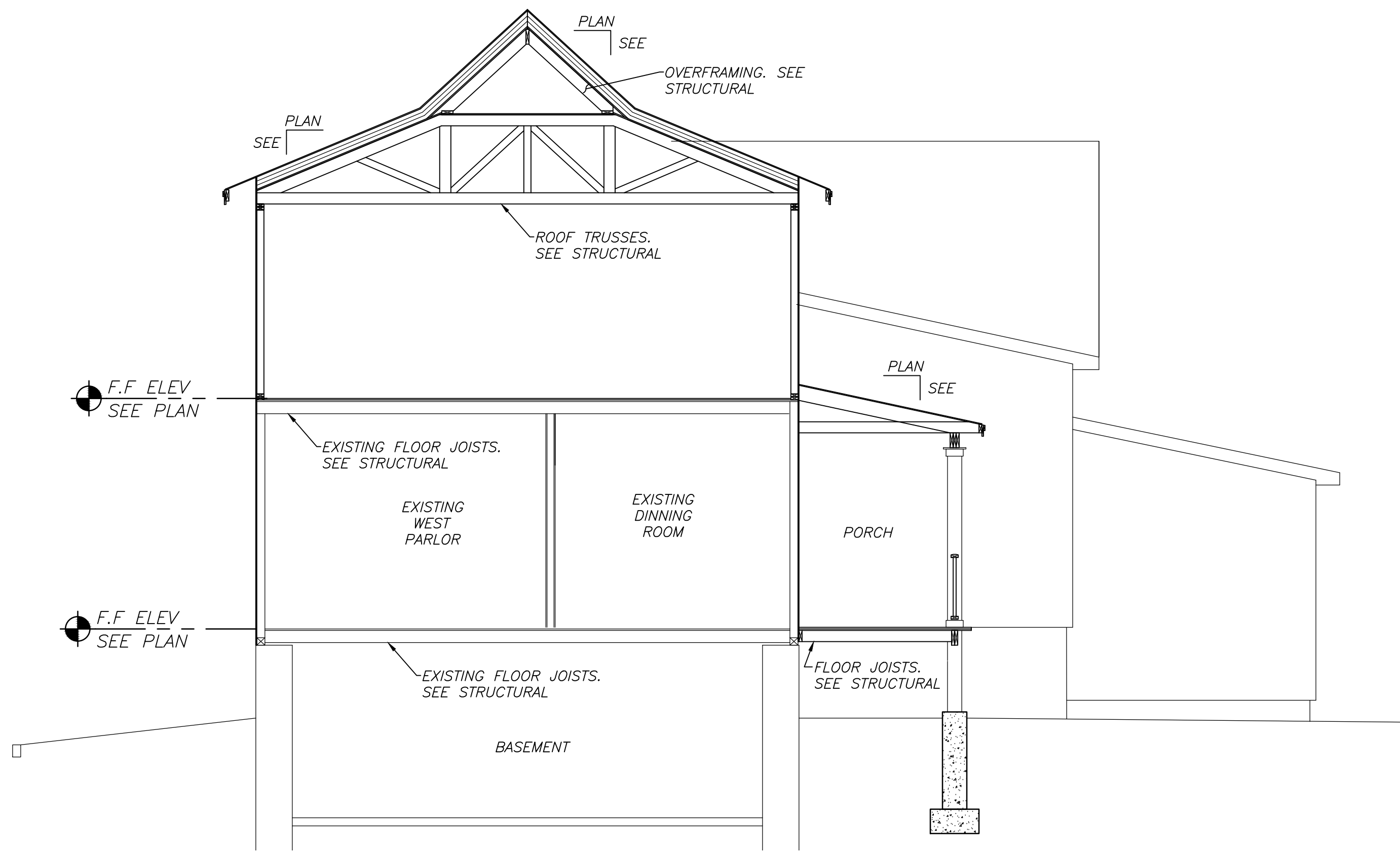
5 SECTION SCALE: 1/4" = 1'-0"
