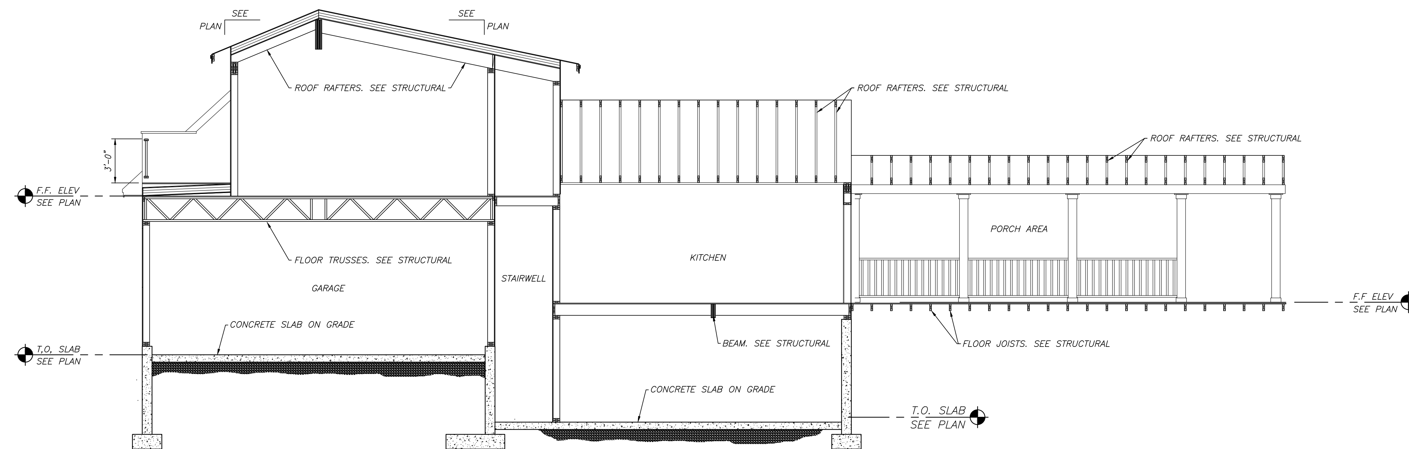
A1 SECTION SCALE: 1/4" = 1'-0"
