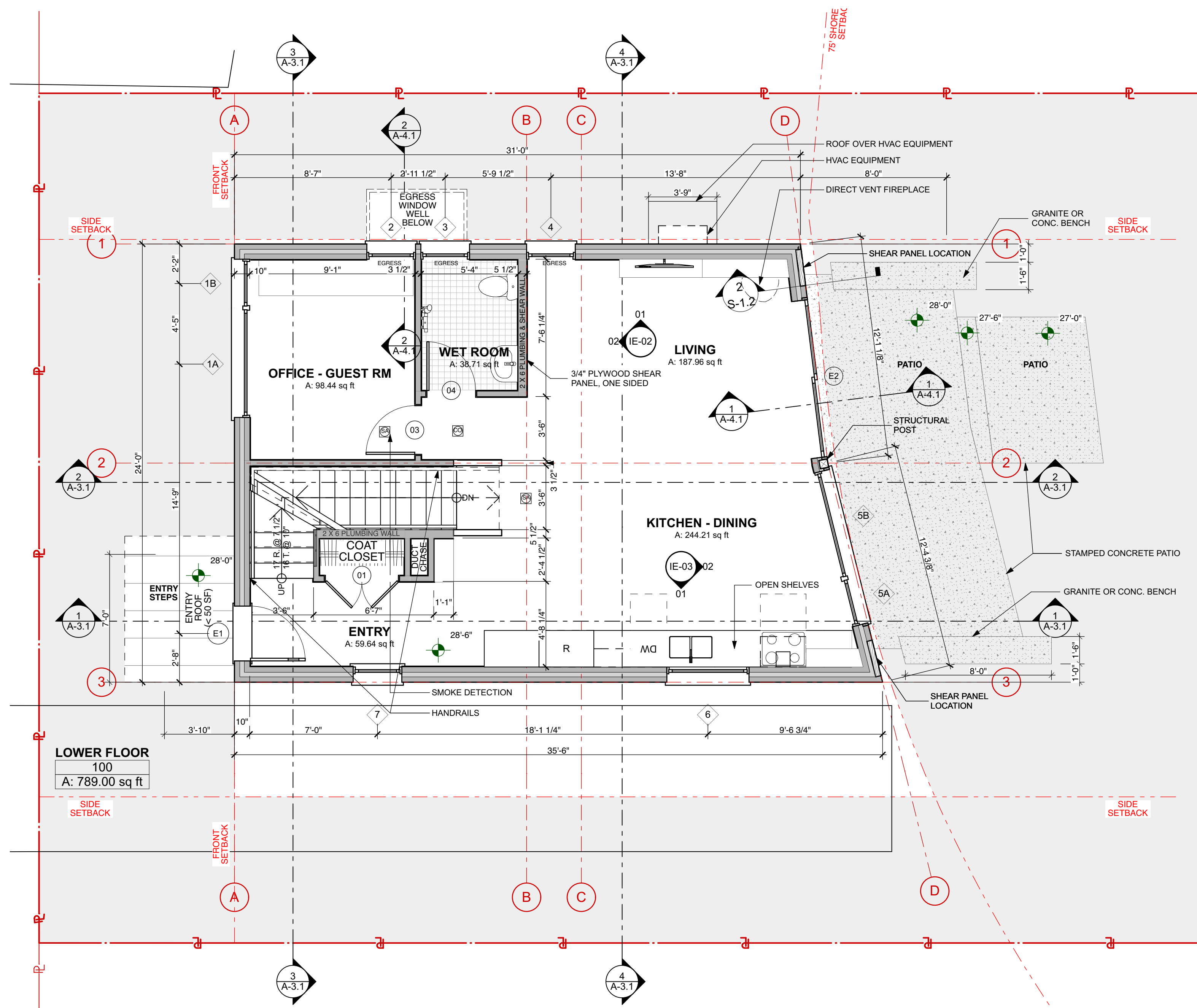
2 MAIN LEVEL SCALE: 1/4" = 1'-0"
