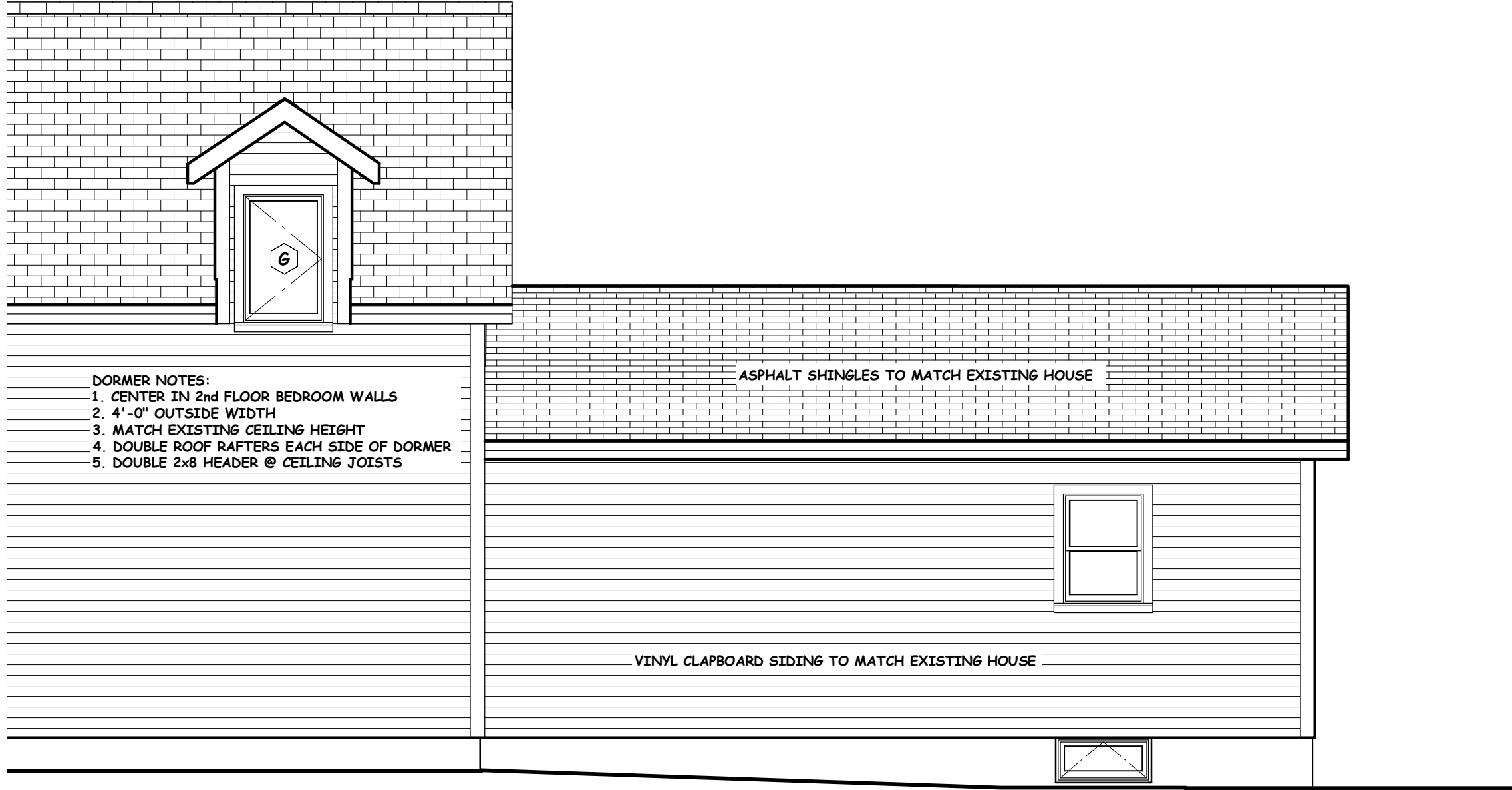
RIGHT ELEVATION
