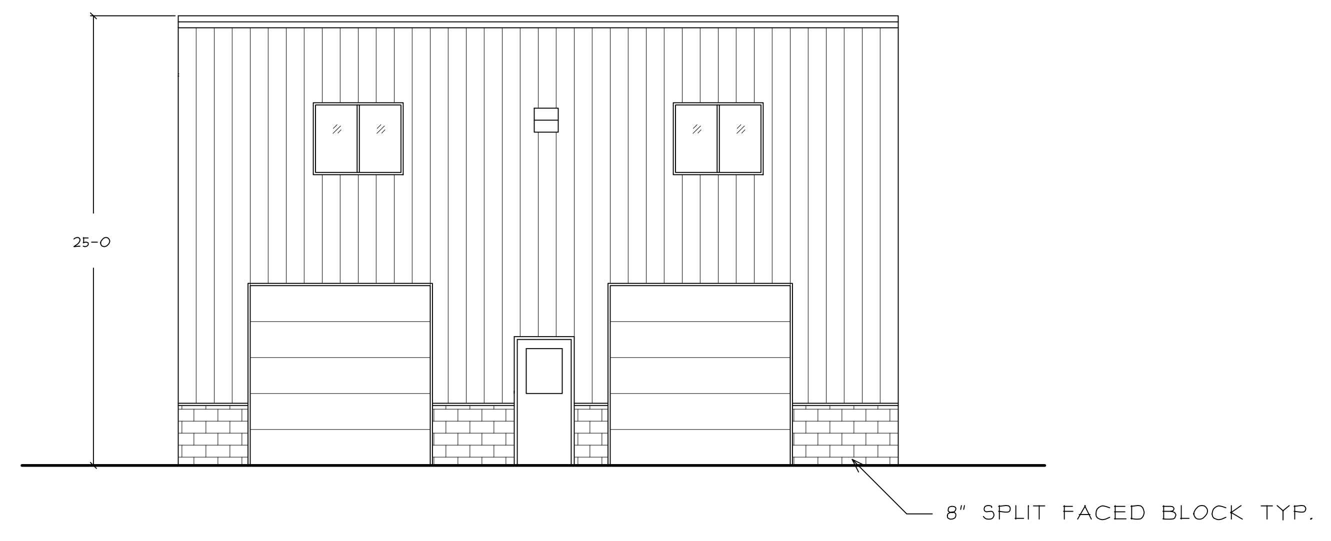
RIGHT ELEVATION
