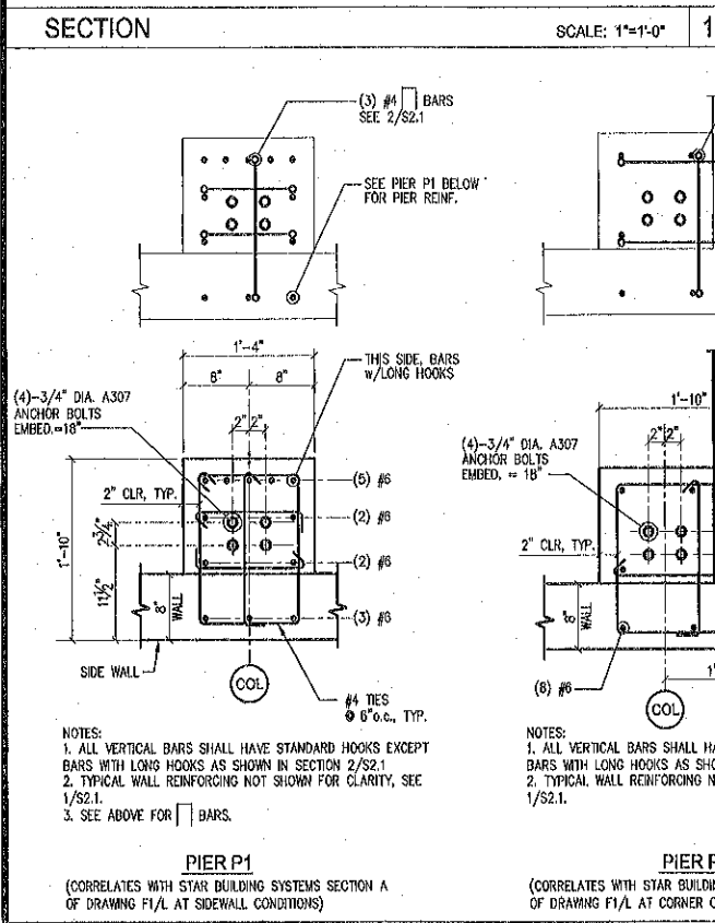
SECTION 1 SCALE: 1"=1'-0"
