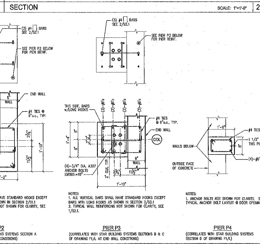
SECTION 2 SCALE: 1"=1'-0"
