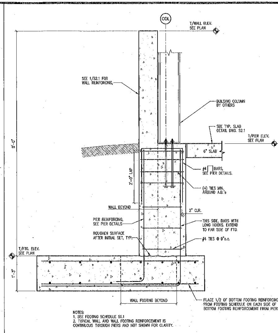
SECTION 2 SCALE: 1"=1'-0"
