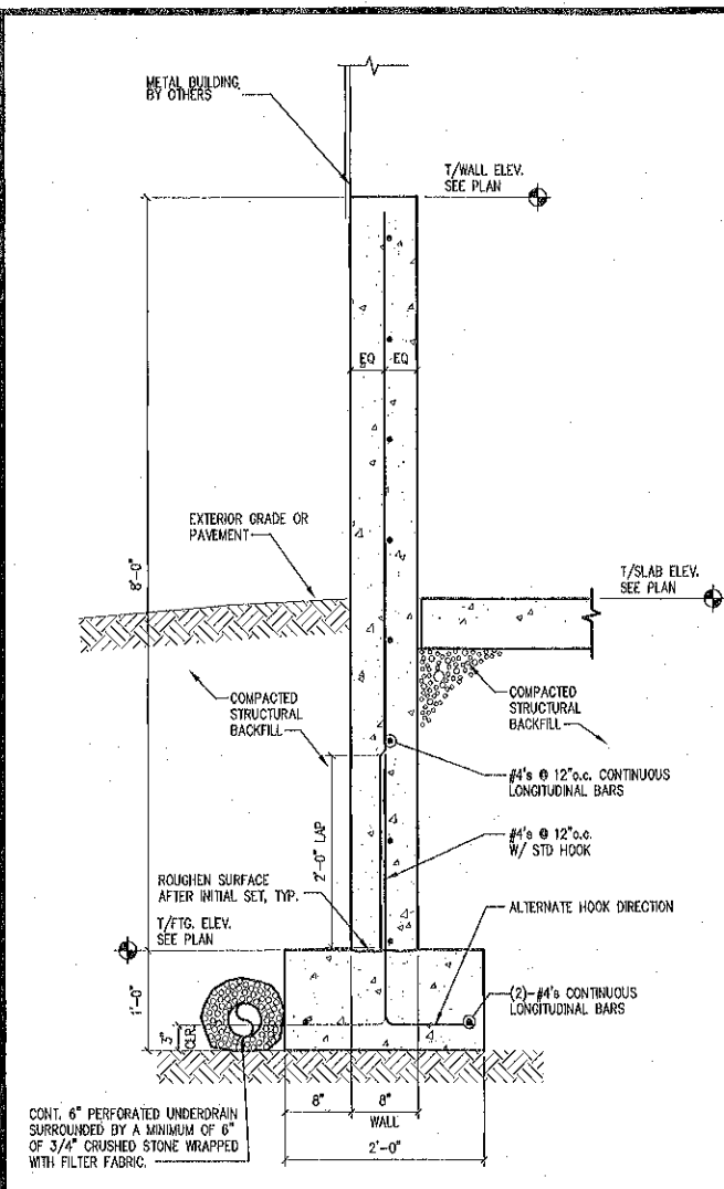
SECTION 1 SCALE: 1"=1'-0"
