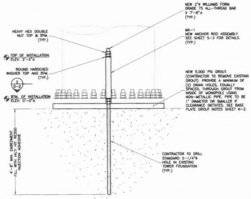
1 S-2 ELEVATION SCALE: 1/2" = 1'-0"
