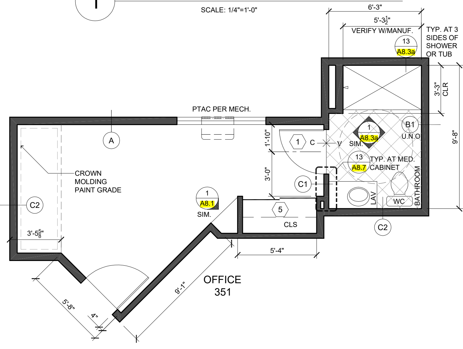
4 OFFICE SCALE: 1/4"=1'-0"
