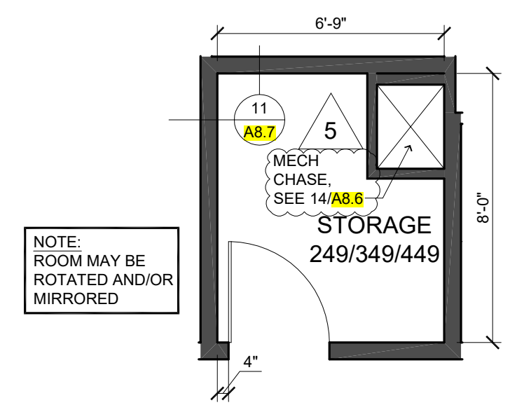
5 STORAGE SCALE: 1/4"=1'-0"
