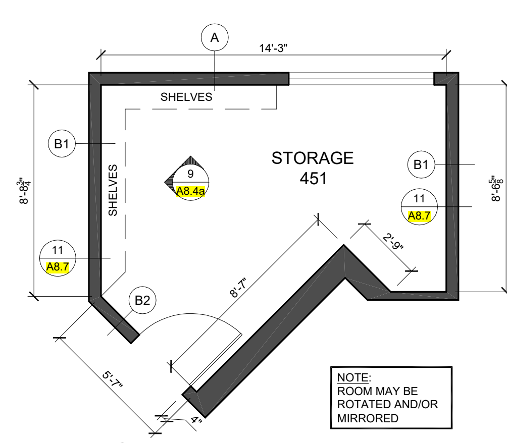
6 STORAGE SCALE: 1/4"=1'-0"
