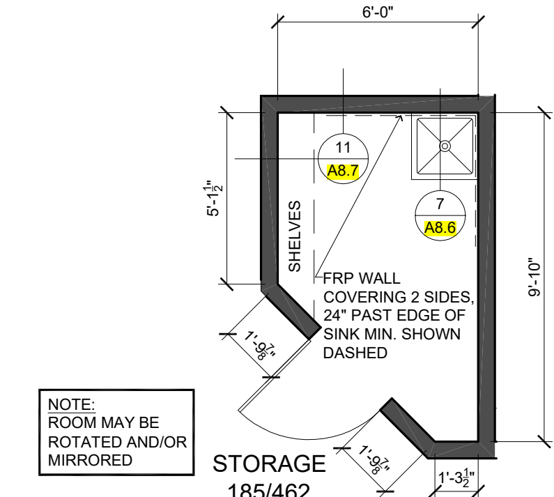
9 STORAGE SCALE: 1/4"=1'-0"
