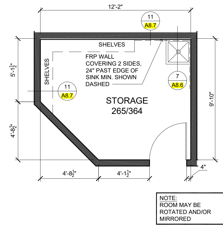
10 STORAGE SCALE: 1/4"=1'-0"
