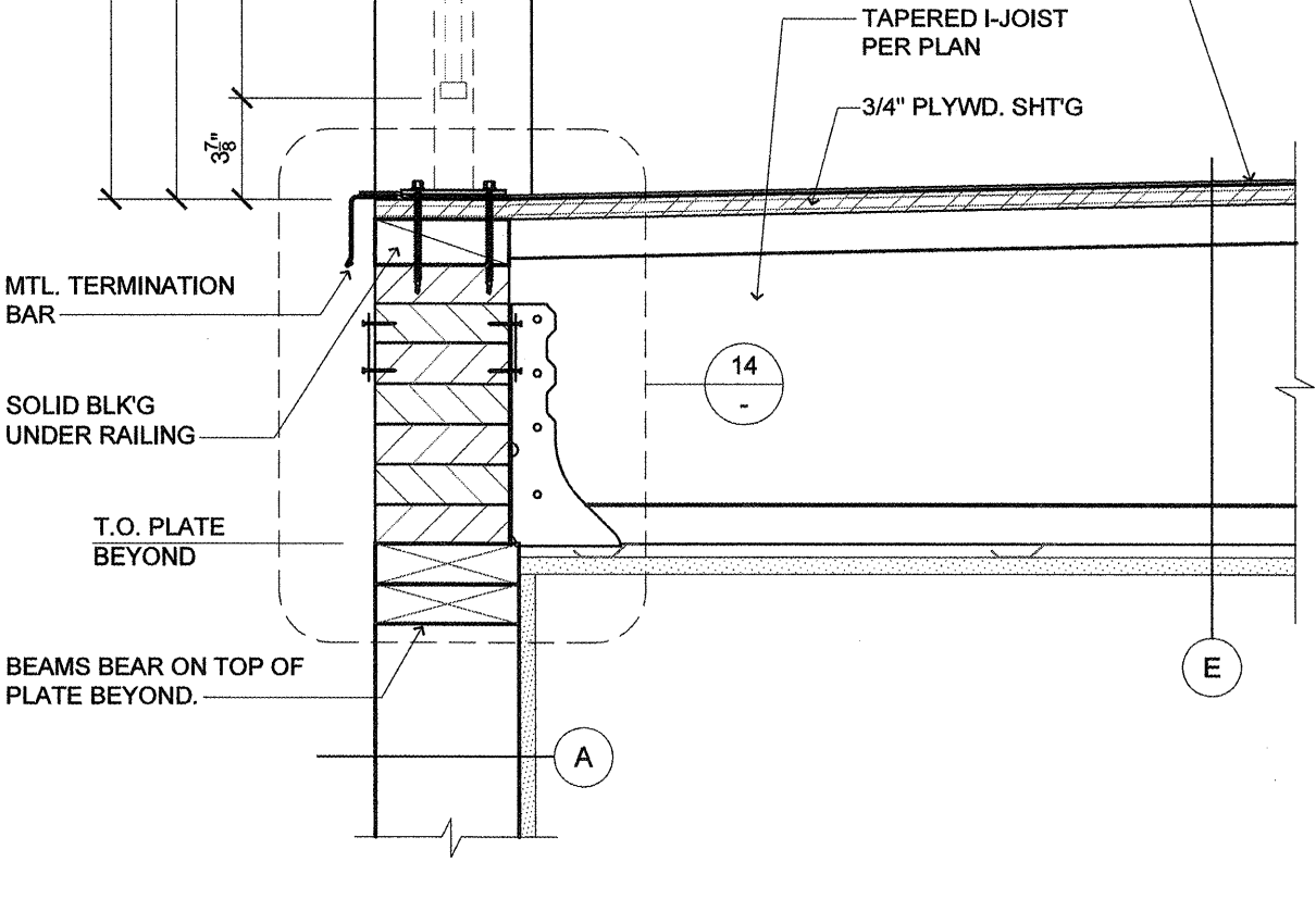
12 DECK DETAIL (DECK EDGE & BEAM) SCALE: 1 1/2" = 1'-0"
