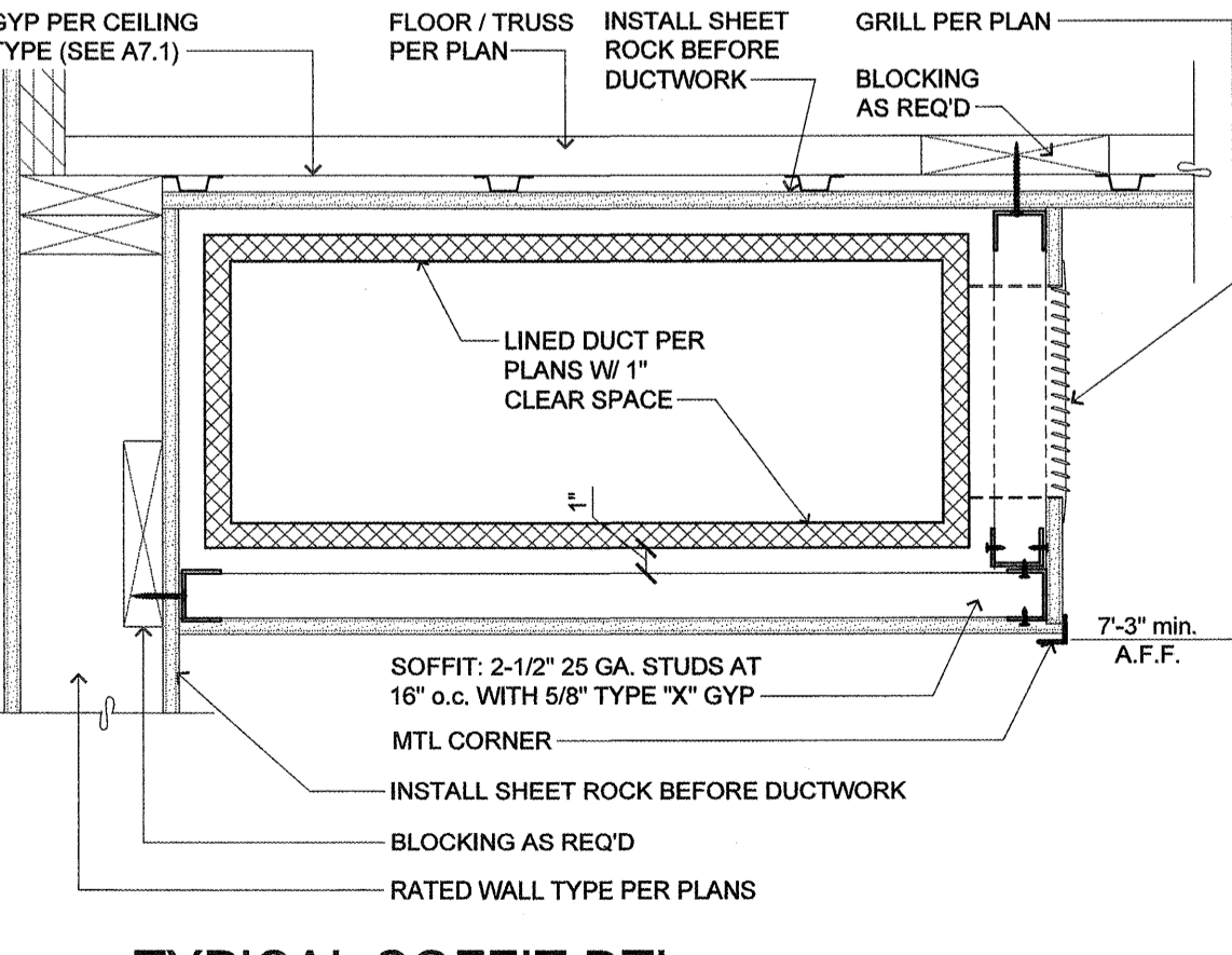
4 TYPICAL SOFFIT DTL. SCALE: 1-1/2" = 1'-0"
