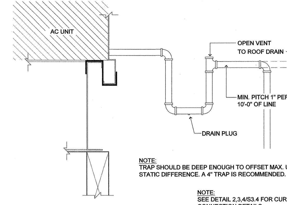
7 ROOFTOP A/C UNIT (TRAP CONDENSATE DRAIN) SCALE: 3"=1'-0"
