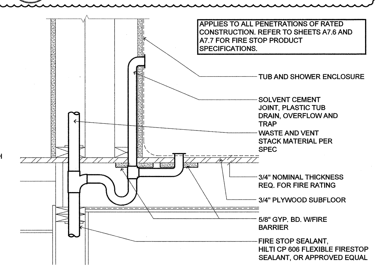
2 TUB AND SHOWER DRAIN DETAIL SCALE: N.T.S.
