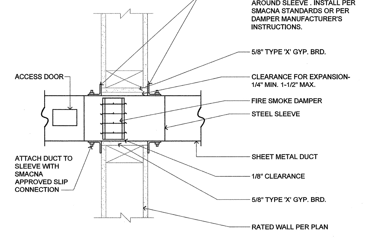
4 FIRE/SMOKE DAMPER IN WALL SCALE: N.T.S.
