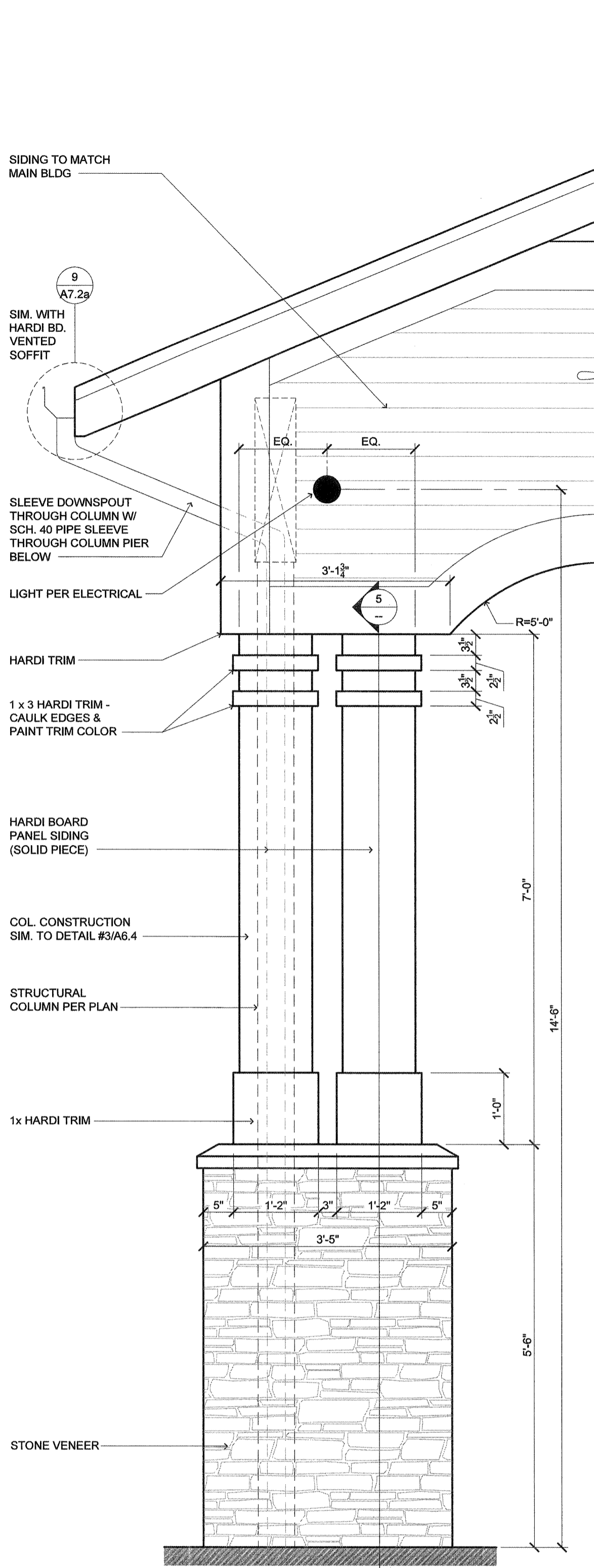
2 PORTE COCHERE SCALE: 3/4" = 1'-0"
