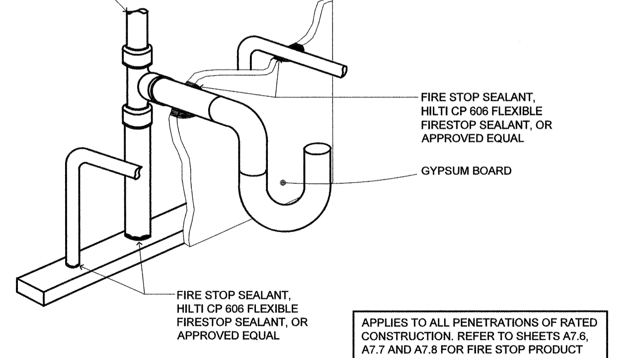
2 TUB AND SHOWER DRAIN DETAIL SCALE: N.T.S.
