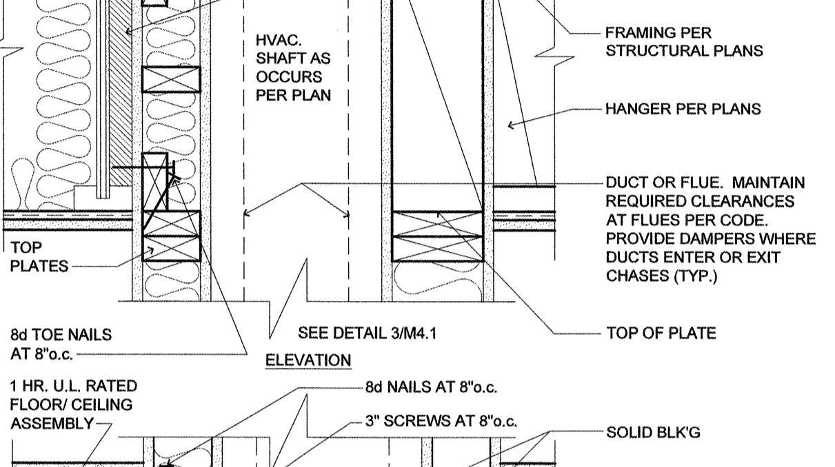
4 FIRE/SMOKE DAMPER IN WALL SCALE: N.T.S.
