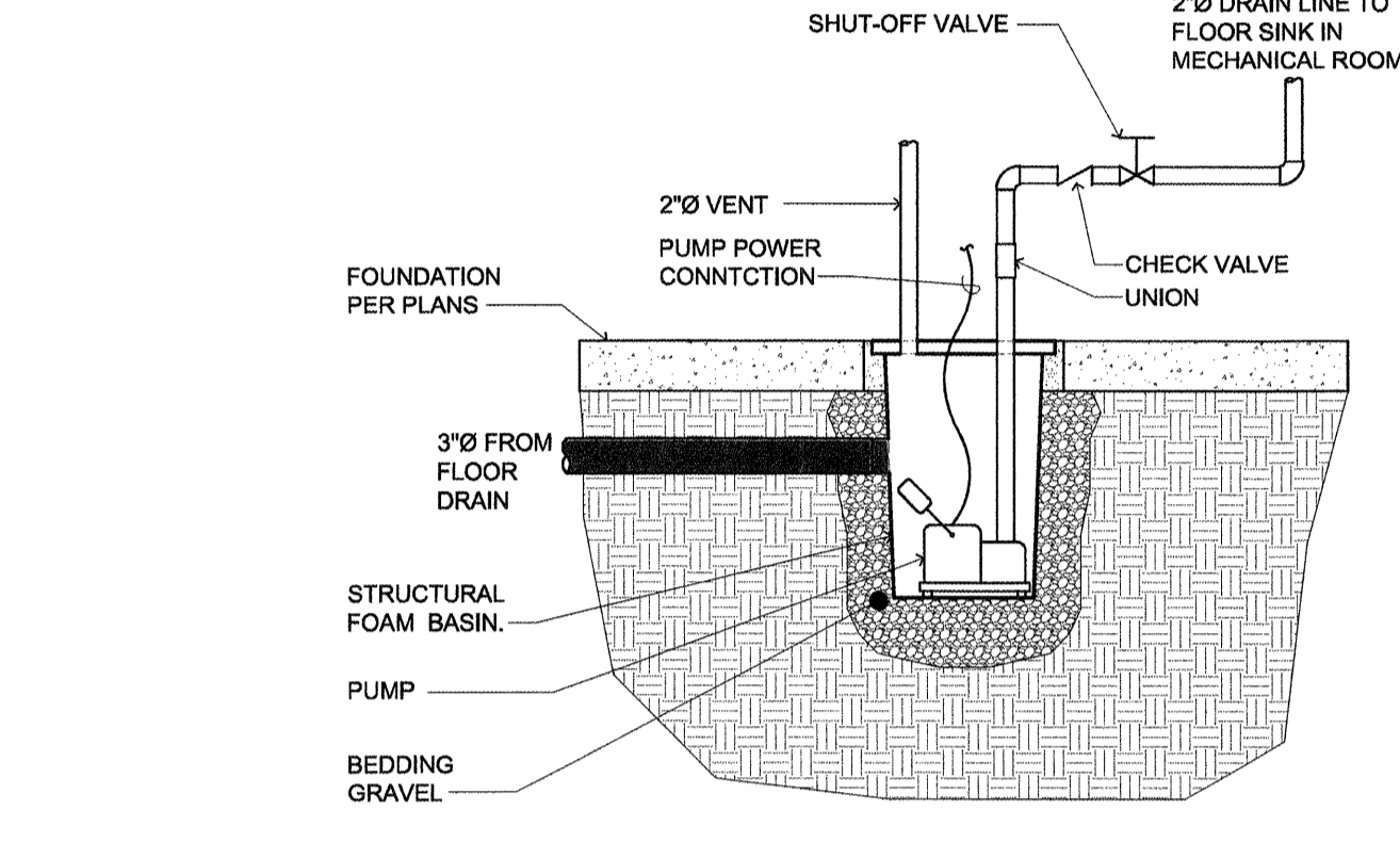
3 SUMP PUMP (P-32) THEATER SCALE: N.T.S.
