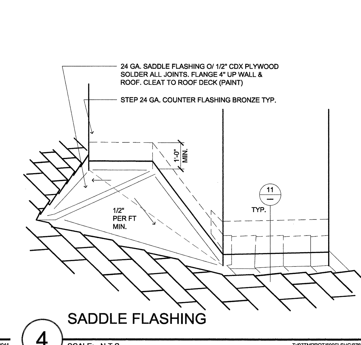
4 SADDLE FLASHING SCALE: N.T.S.
