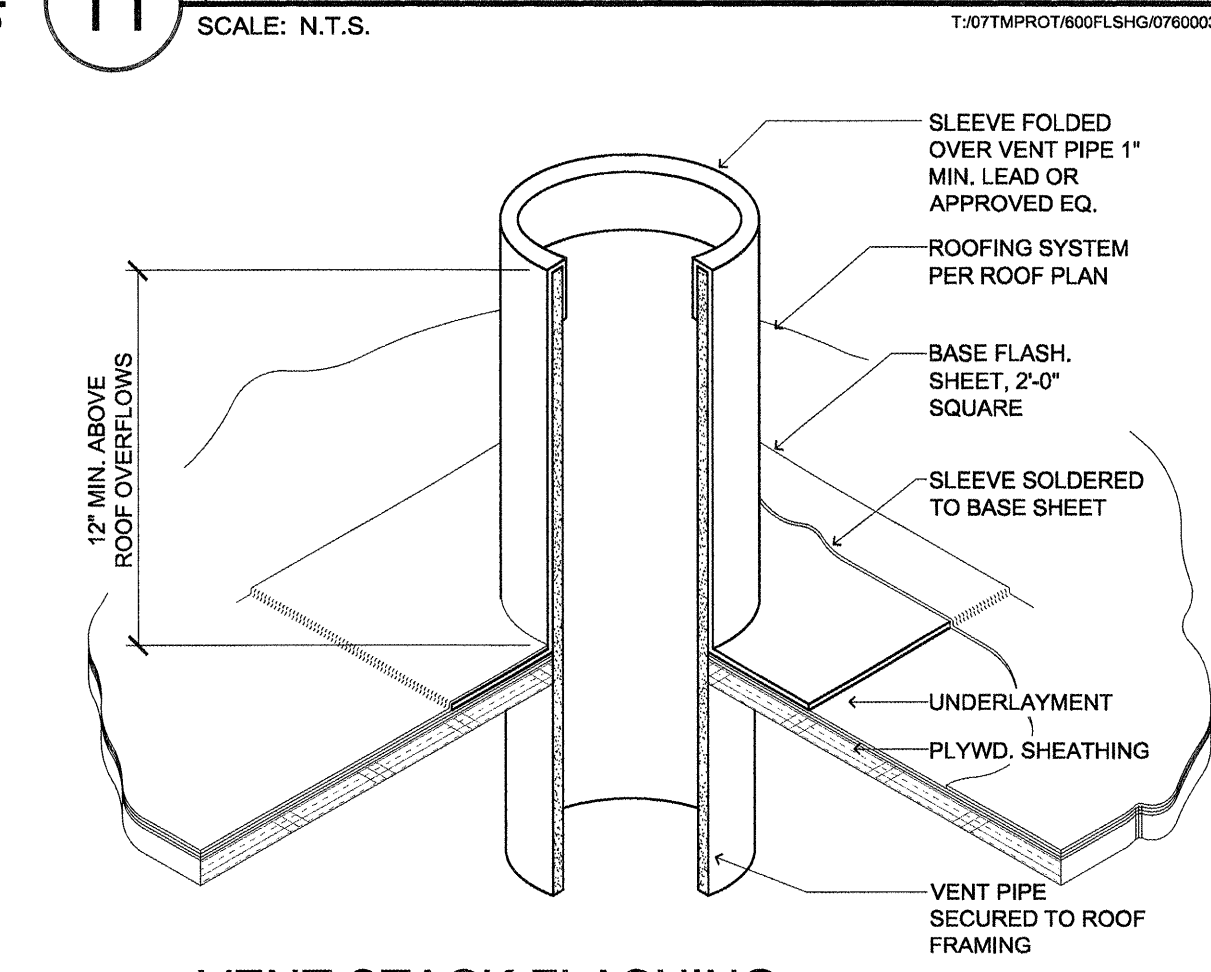
10 VENT STACK FLASHING SCALE: N.T.S.
