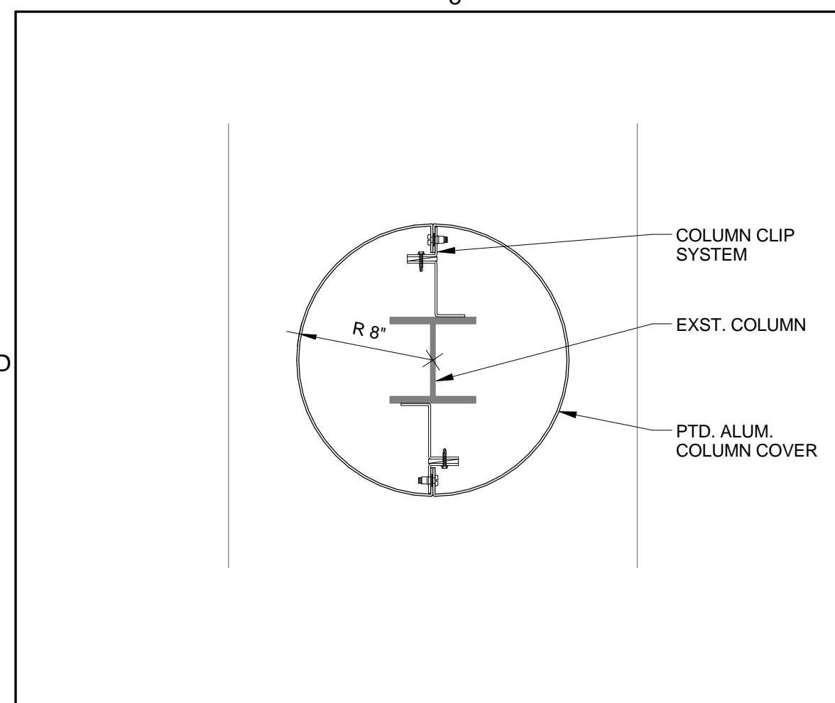
D5 EXTERIOR COLUMN WRAP 1 1/2" = 1'-0"
