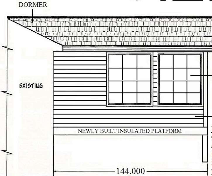
A-WALL ELEVATION
