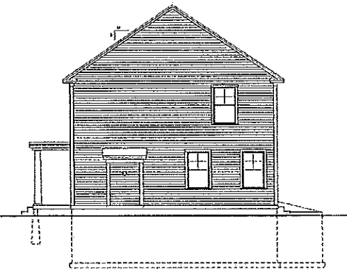
RIGHT ELEVATION
