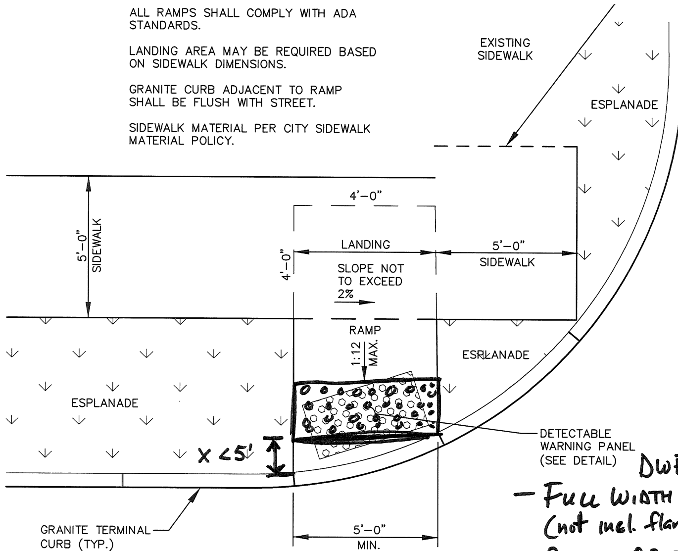
SIDEWALK LAYOUT DETAIL N.T.S.
