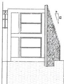
RIGHT ELEVATION
