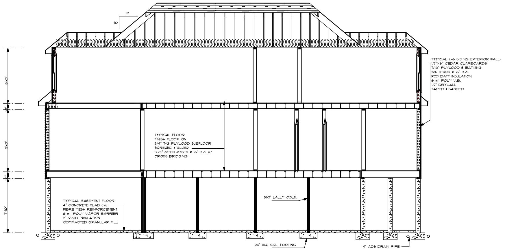
CROSS SECTION A-A SCALE: 1/4" = 1'-0"
