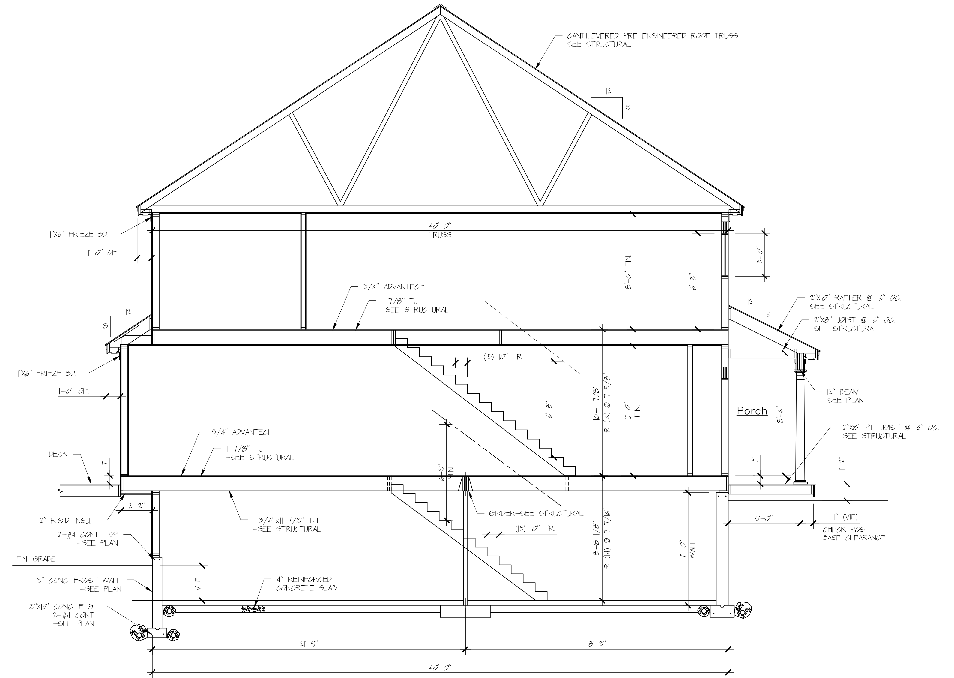
SECTION SCALE: 1/4" = 1'-0"
