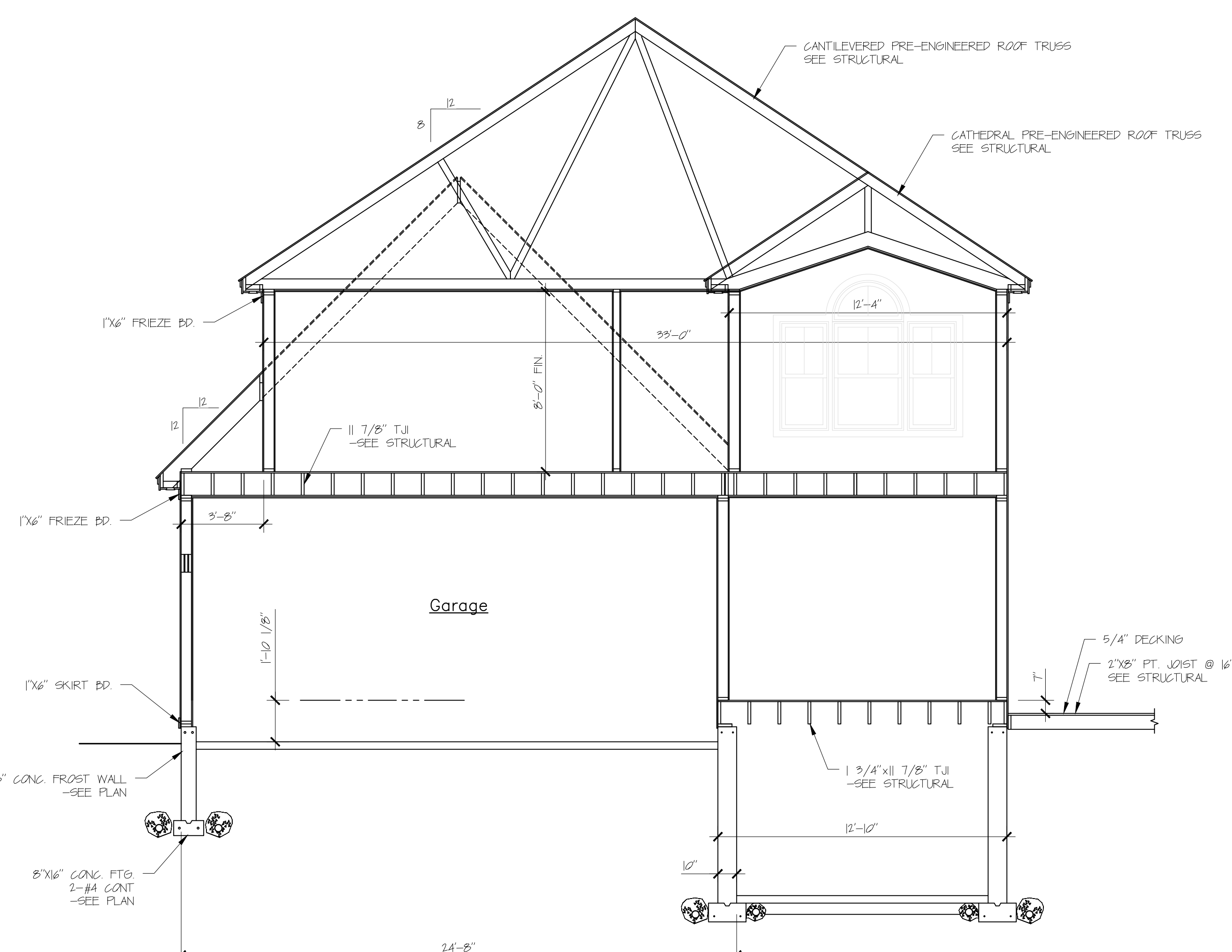
SECTION SCALE: 1/4" = 1'-0"
