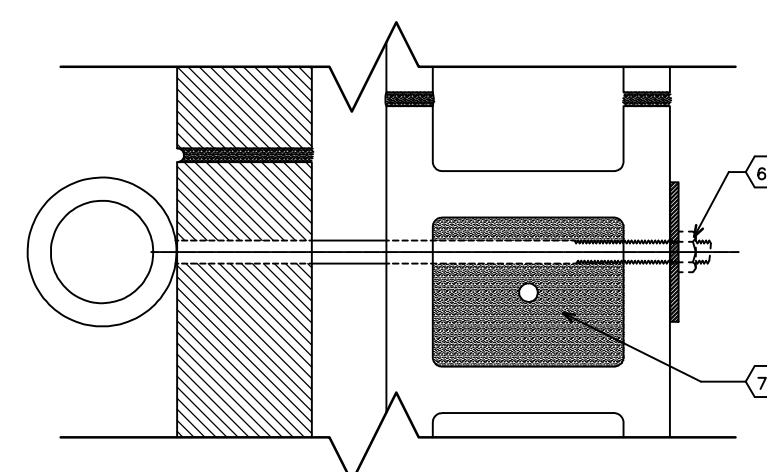
PLAN/SECTION - EYEBOLT N.T.S.
