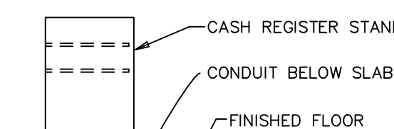
2 DETAIL N.T.S.
