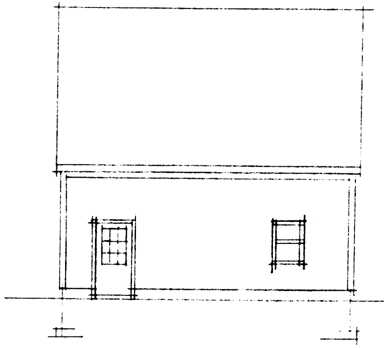
RIGHT ELEVATION
