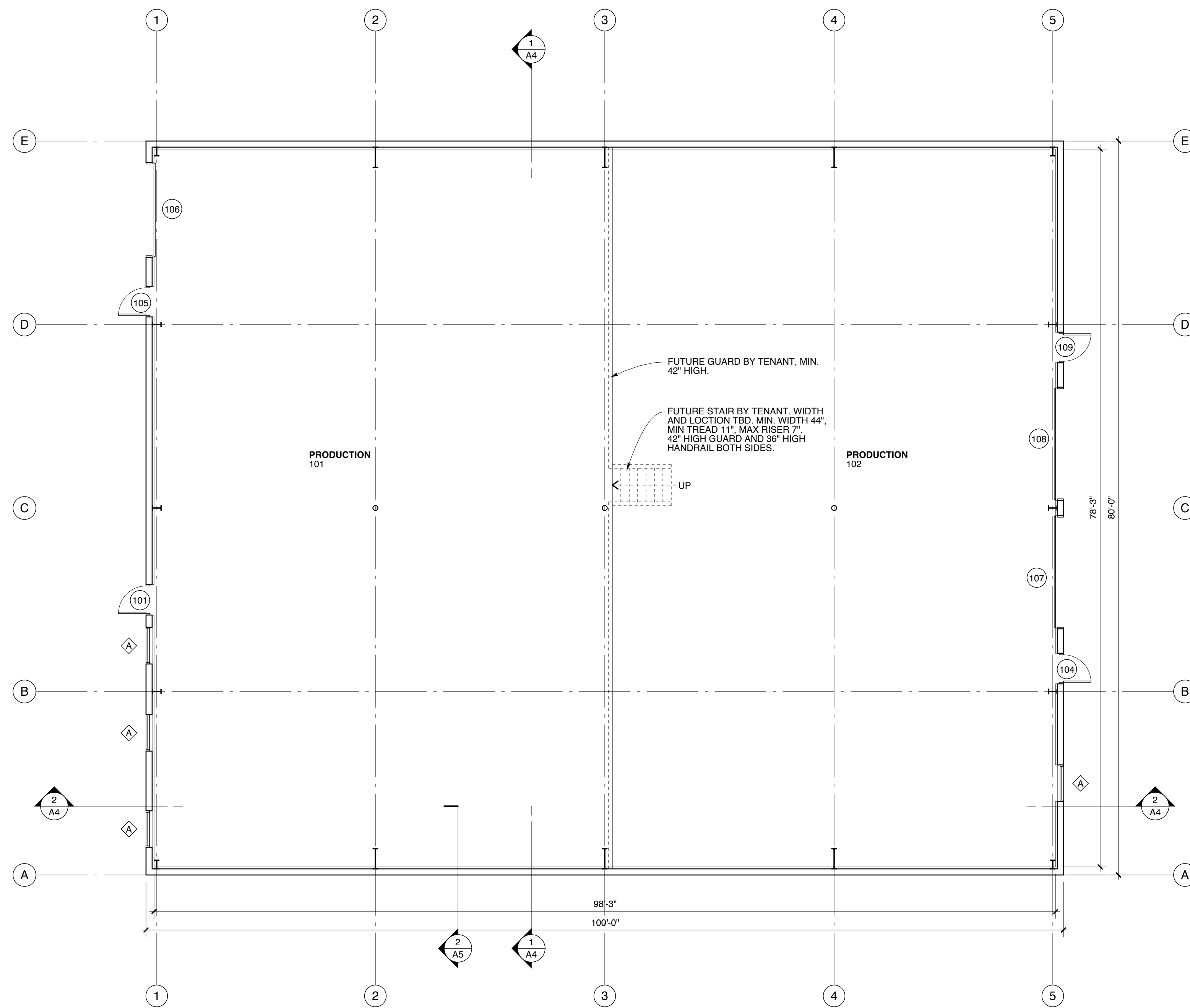
1 FLOOR PLAN SCALE: 1/8" = 1'-0"
