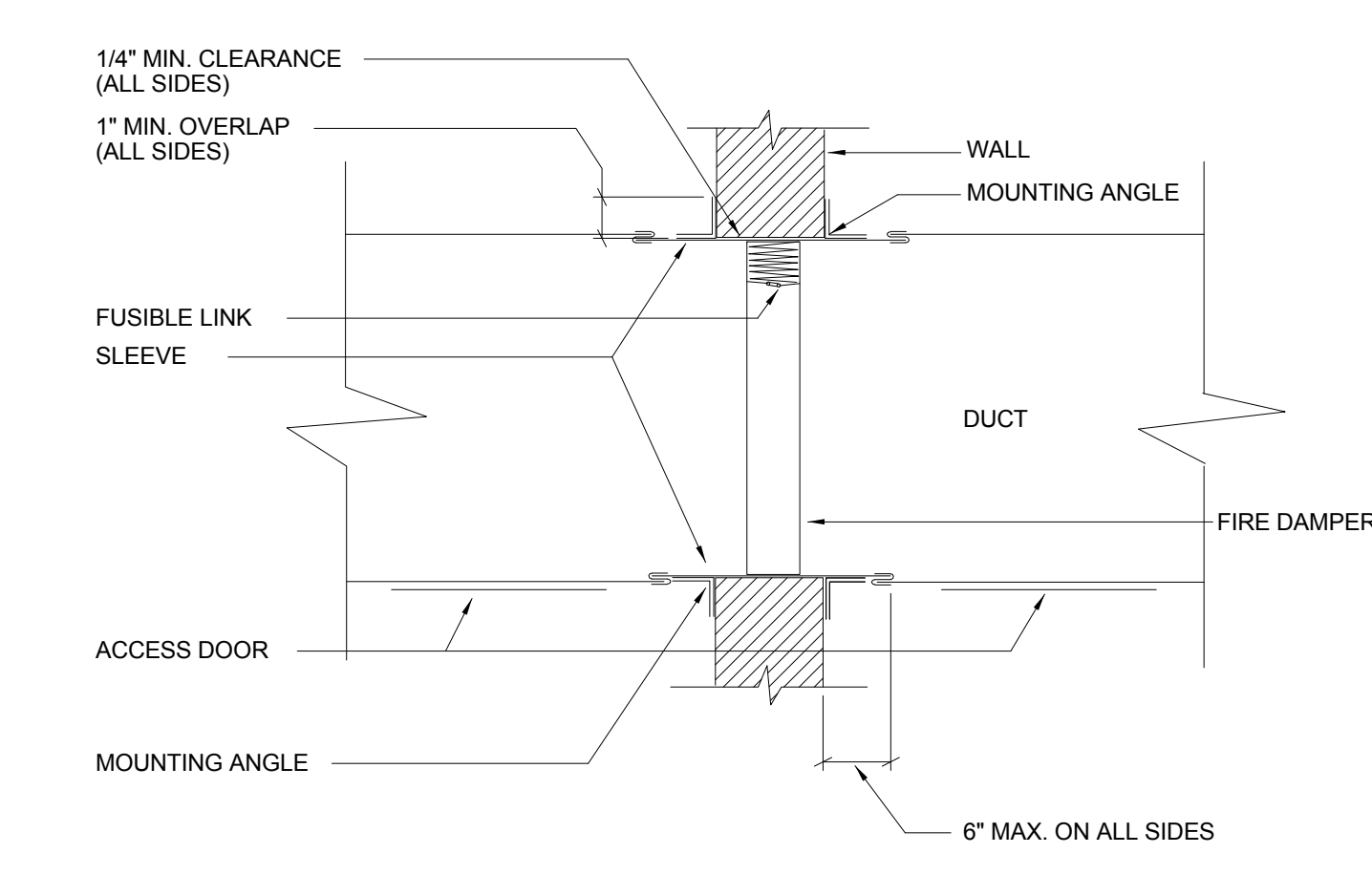
14 FIRE DAMPER DETAIL MH-801-C N.T.S.
