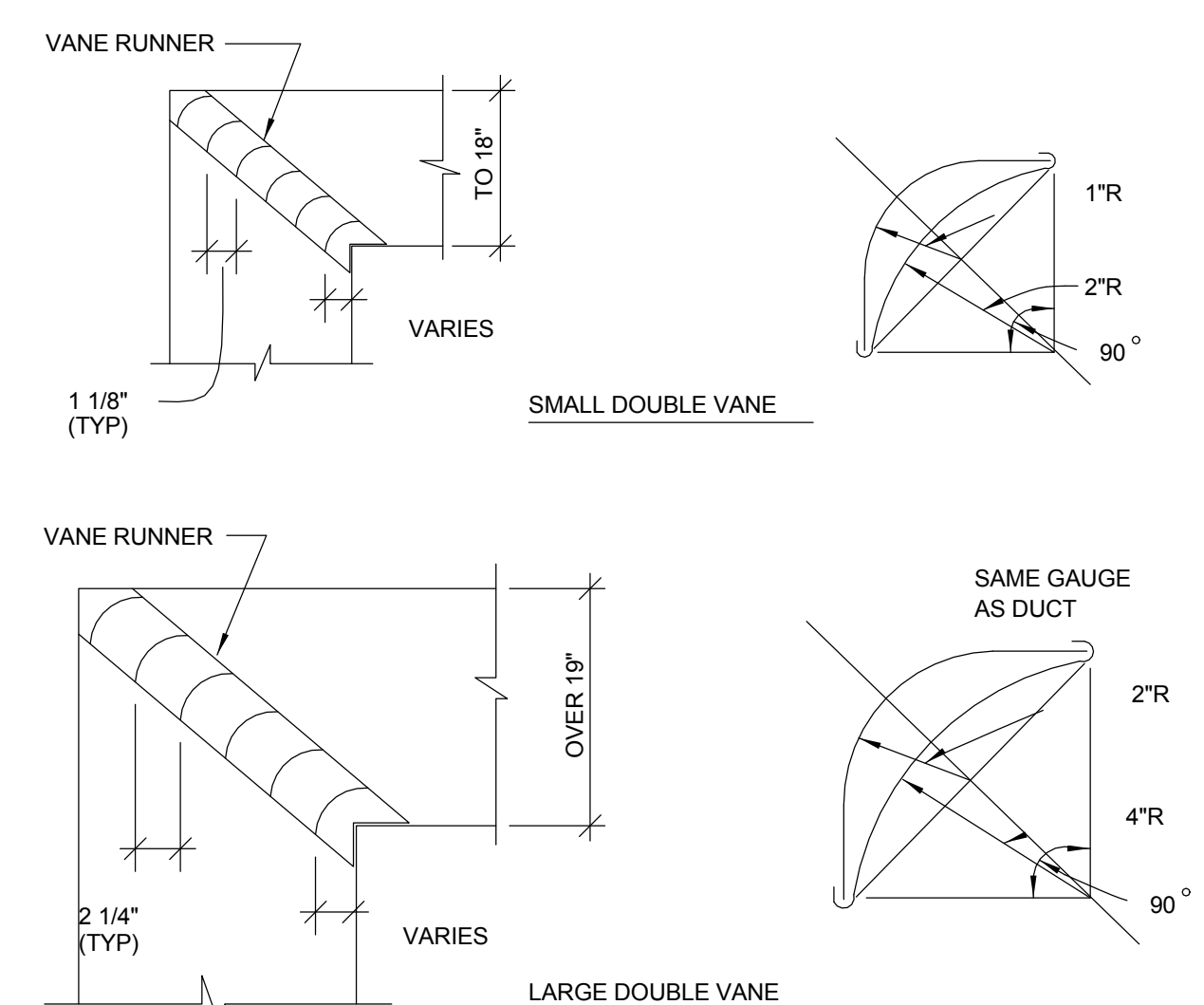
2 DUCT-TURN INSTALLATION DETAIL MH-801-C N.T.S.
