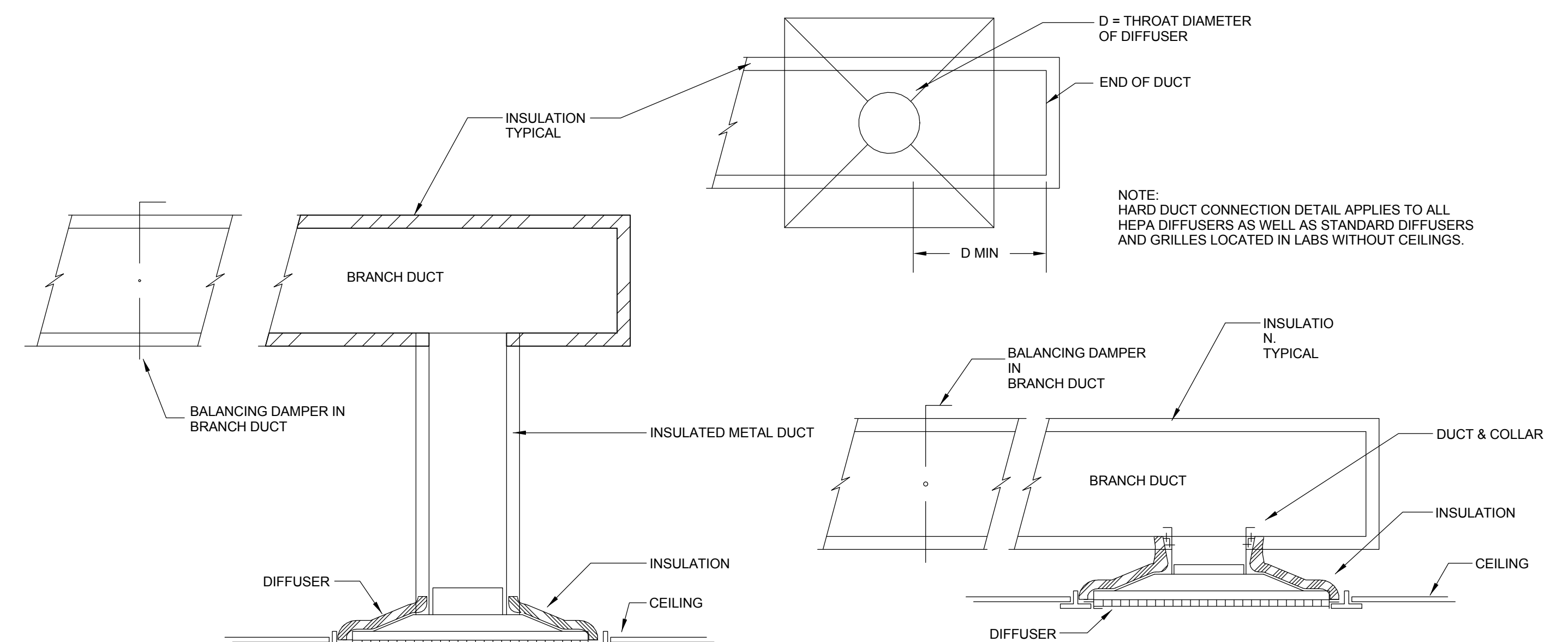
6 SUPPLY AIR DIFFUSER DETAIL MH-801-C N.T.S.
