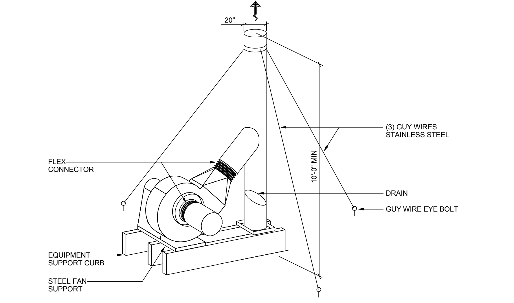
13 EXHAUST FAN DETAIL MH-801-C N.T.S.
