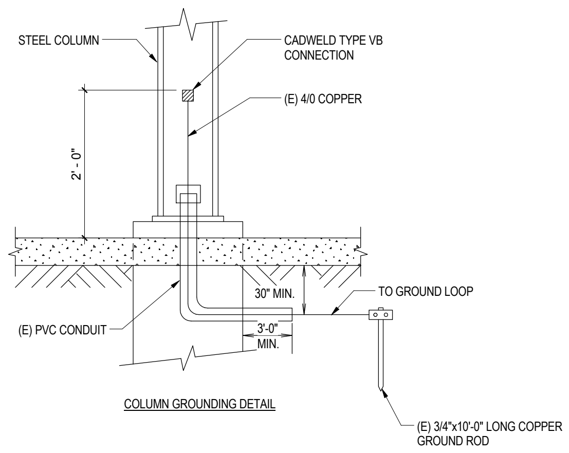
1 PHASE B - GROUNDING DETAILS E-801-B N.T.S.
