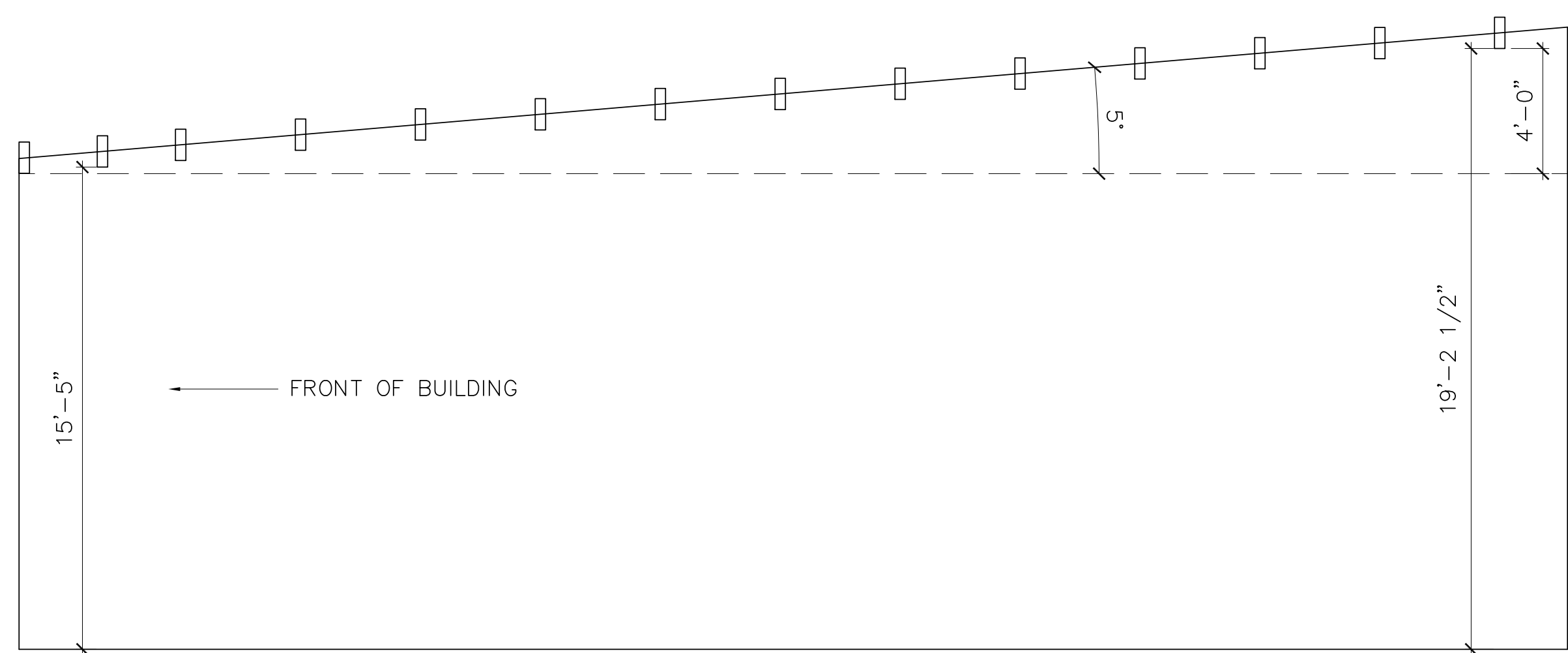
ELEVATION
