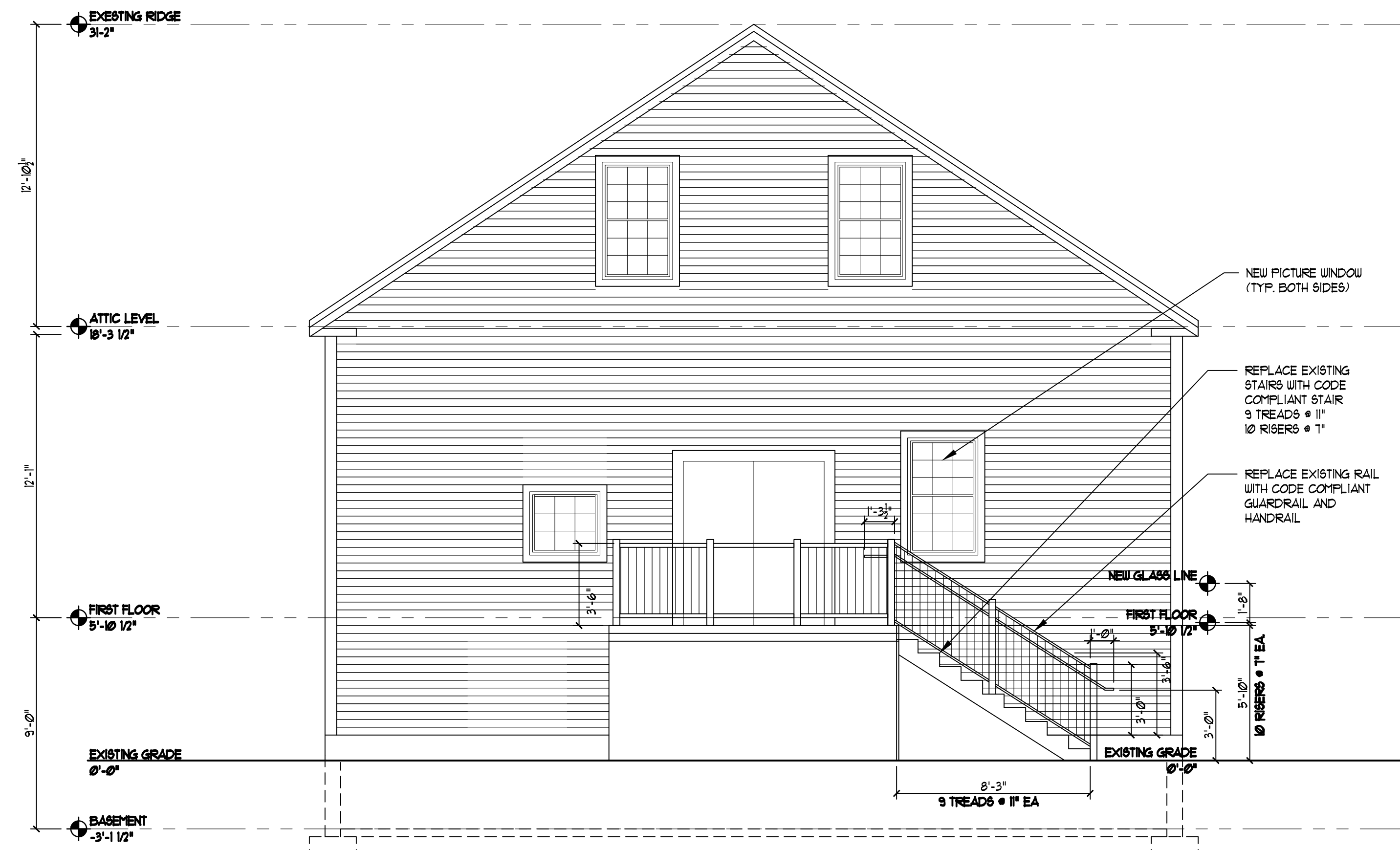
1 NORTH ELEVATION A3 SCALE: 1/4" = 1'-0"
