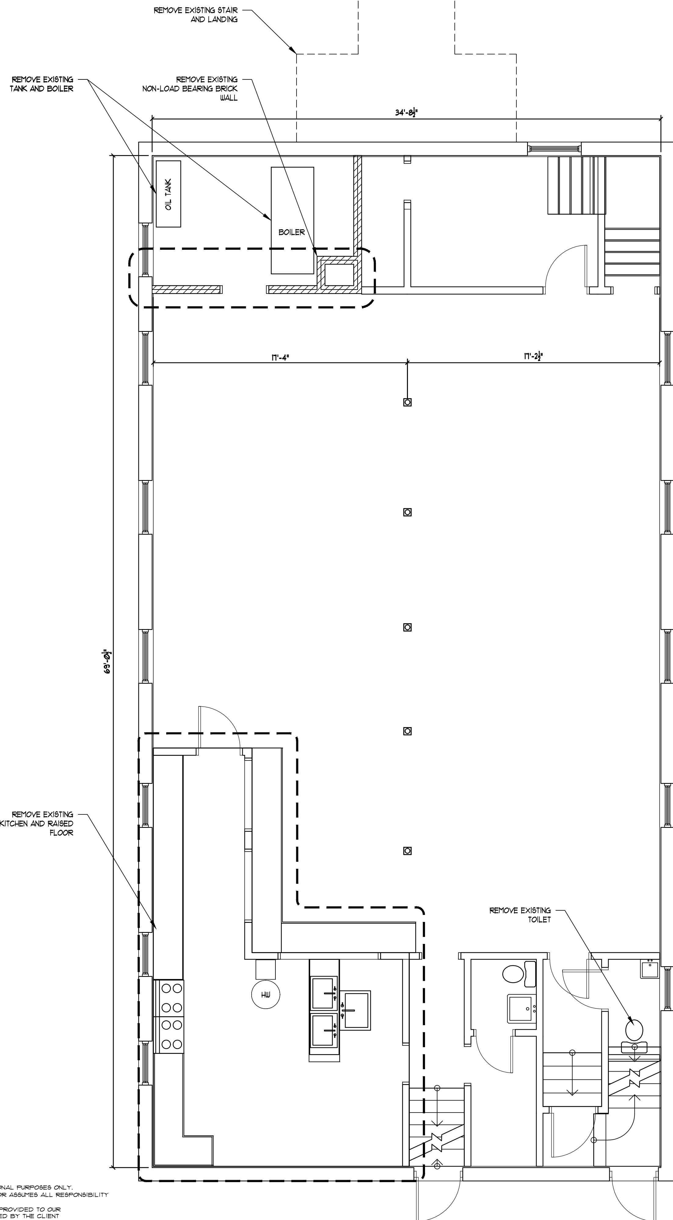
1 BASEMENT DEMO PLAN D1 SCALE: 1/4" = 1'-0"
