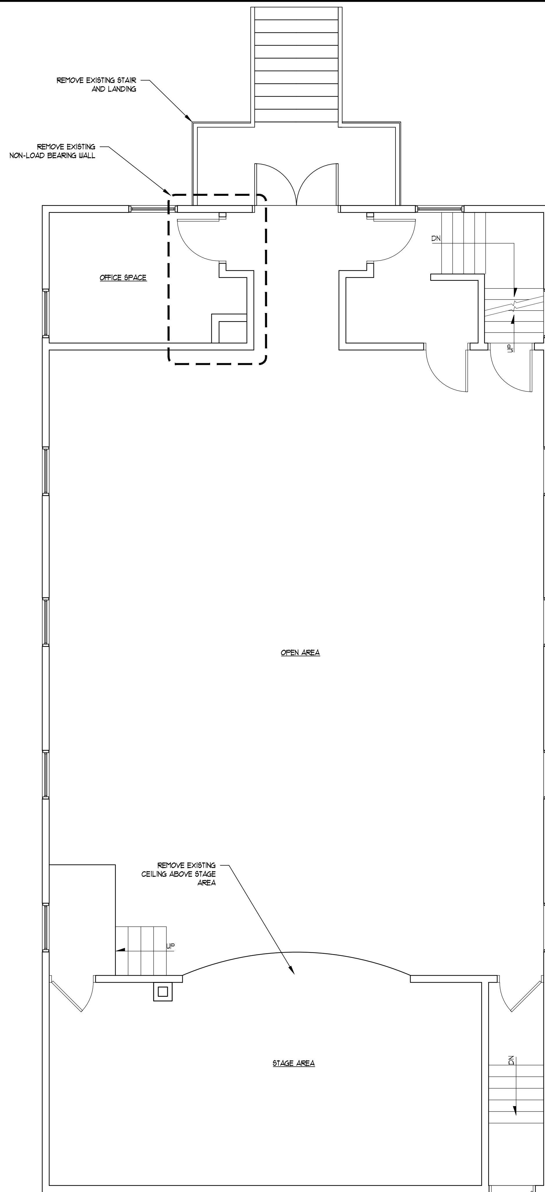
2 FIRST FLOOR DEMO PLAN D1 SCALE: 1/4" = 1'-0"
