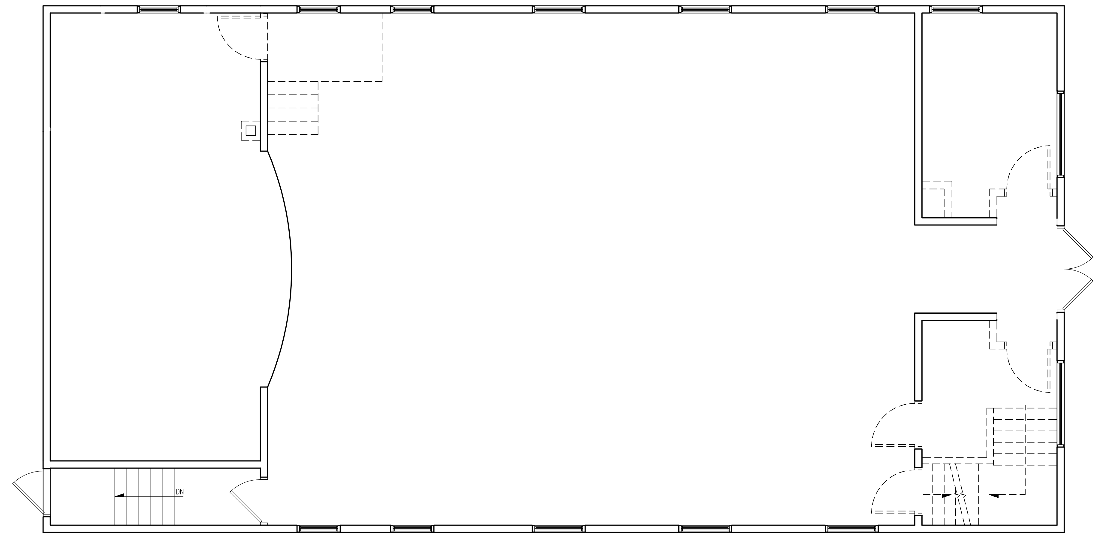
2 FIRST FLOOR DEMO PLAN D1 SCALE: 1/4" = 1'-0"
