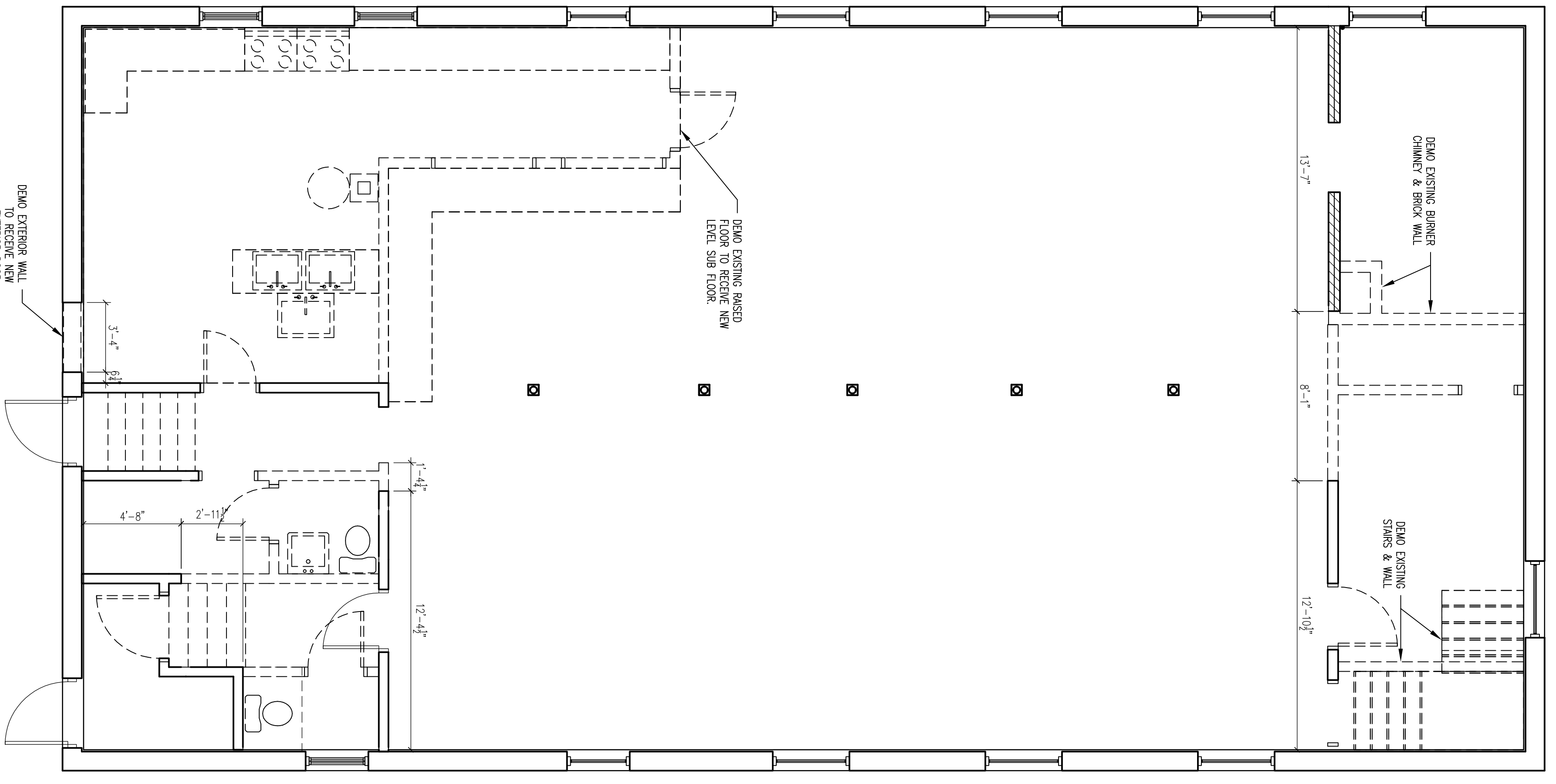
1 BASEMENT DEMO PLAN D1 SCALE: 1/4" = 1'-0"
