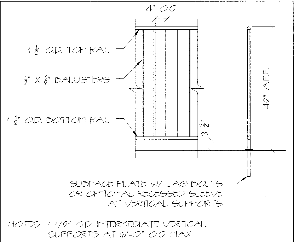
3 TYPICAL EXTERIOR GUARDRAIL N.T.S.
