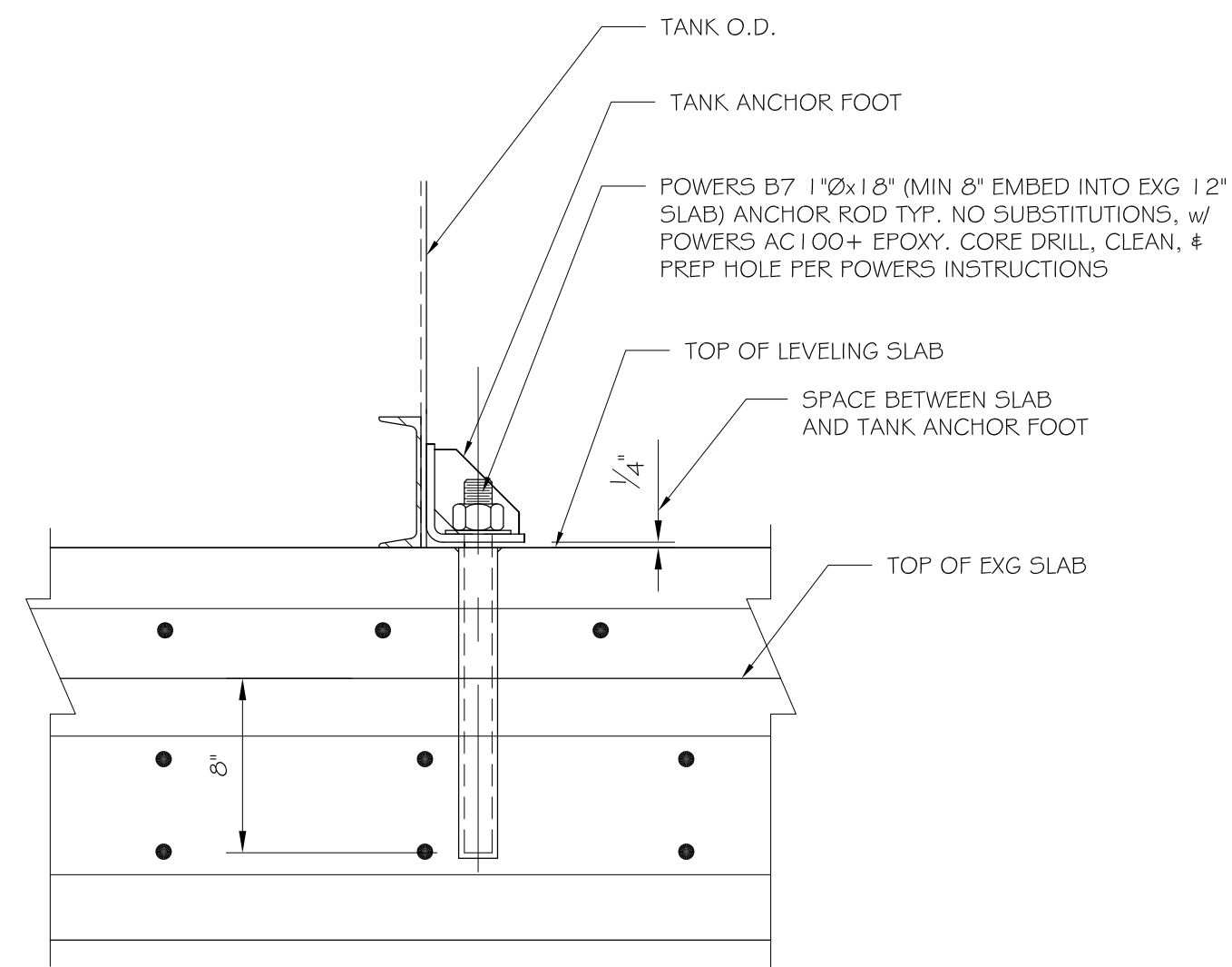
C4 TANK ANCHORS SCALE: 1 1/2" = 1'-0"
