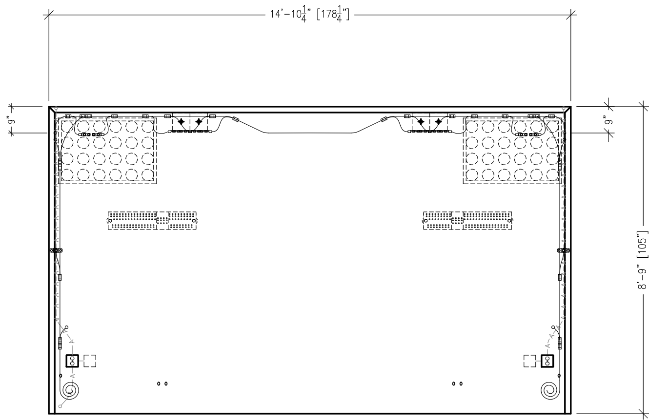
ELEVATION "C"
