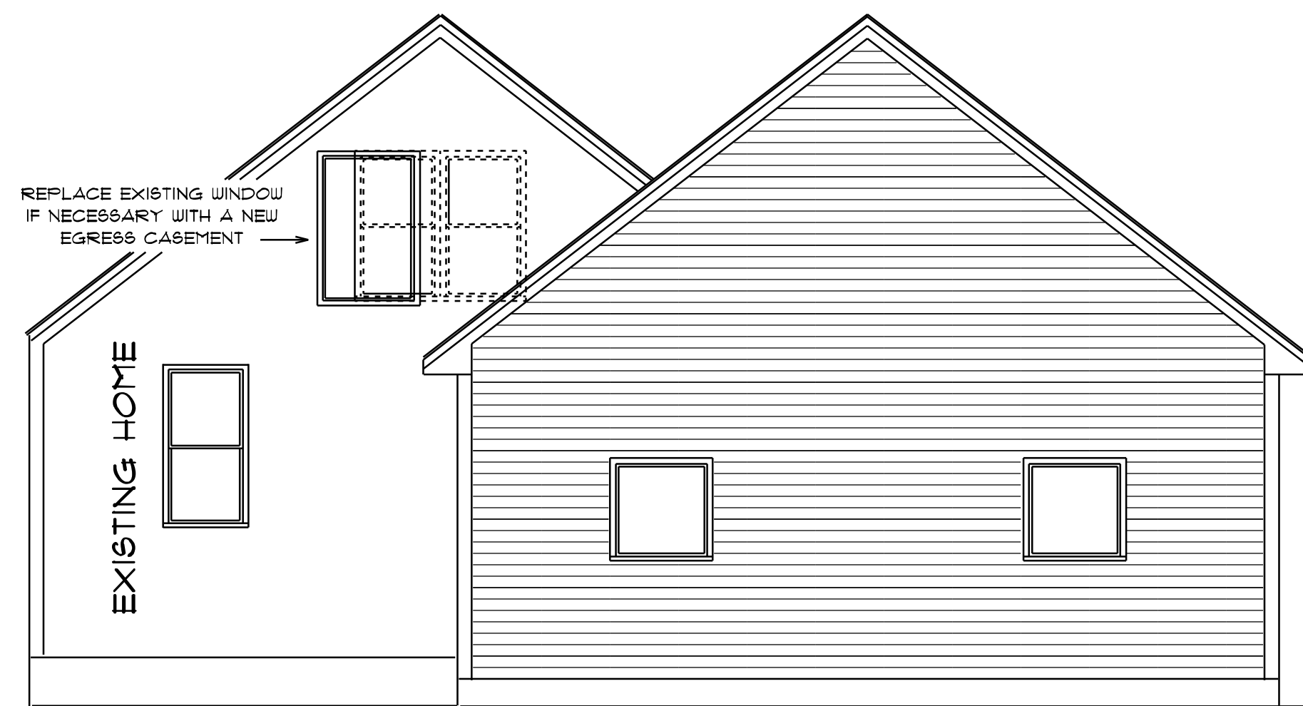
RIGHT ELEVATION
