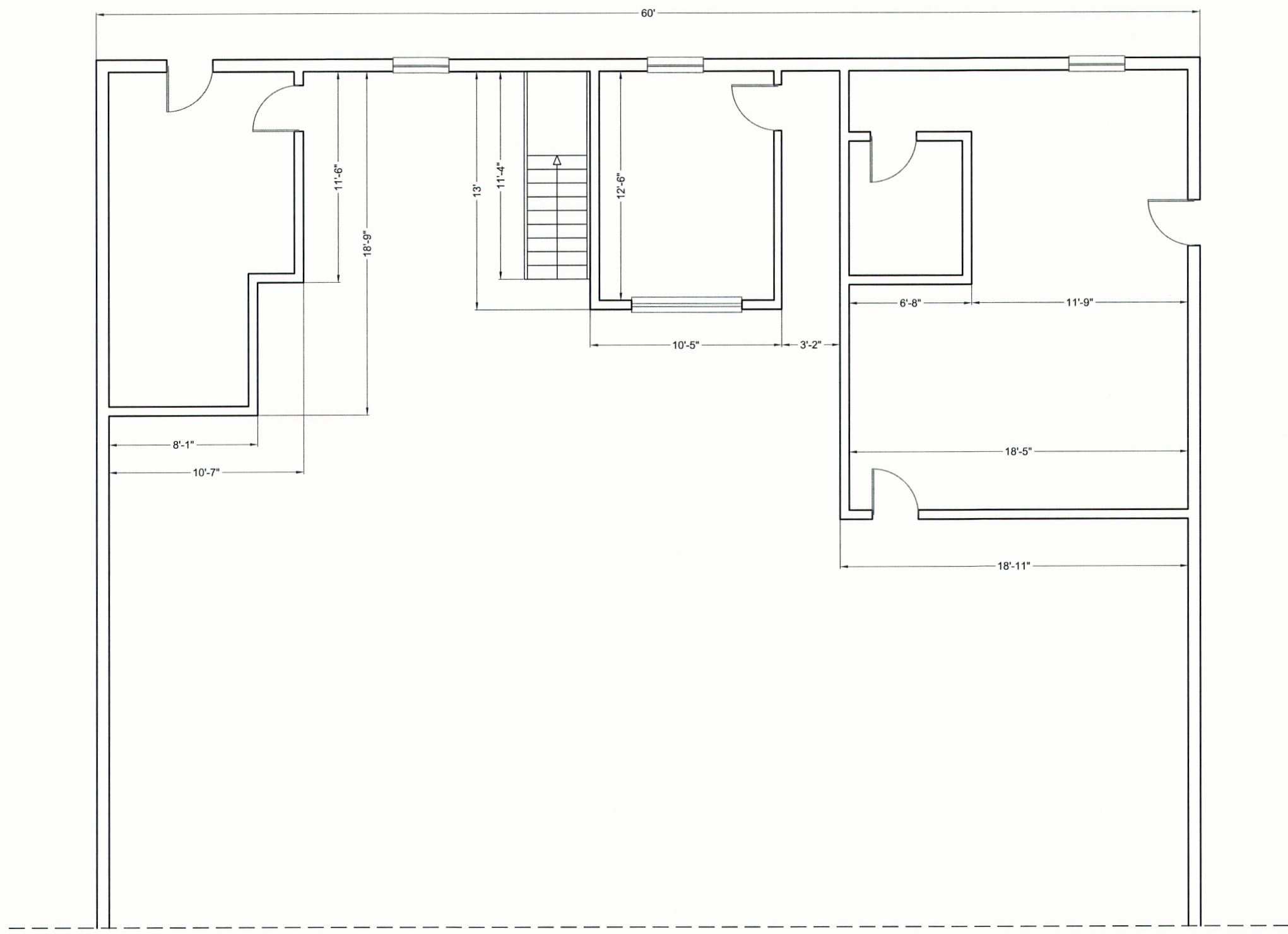
01 New Layout Scale: 1/4" = 1'-0"
