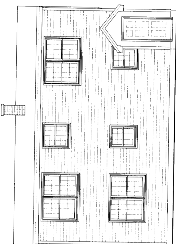
1 REAR ELEVATION A1 SCALE: 1/4"=1'-0"
