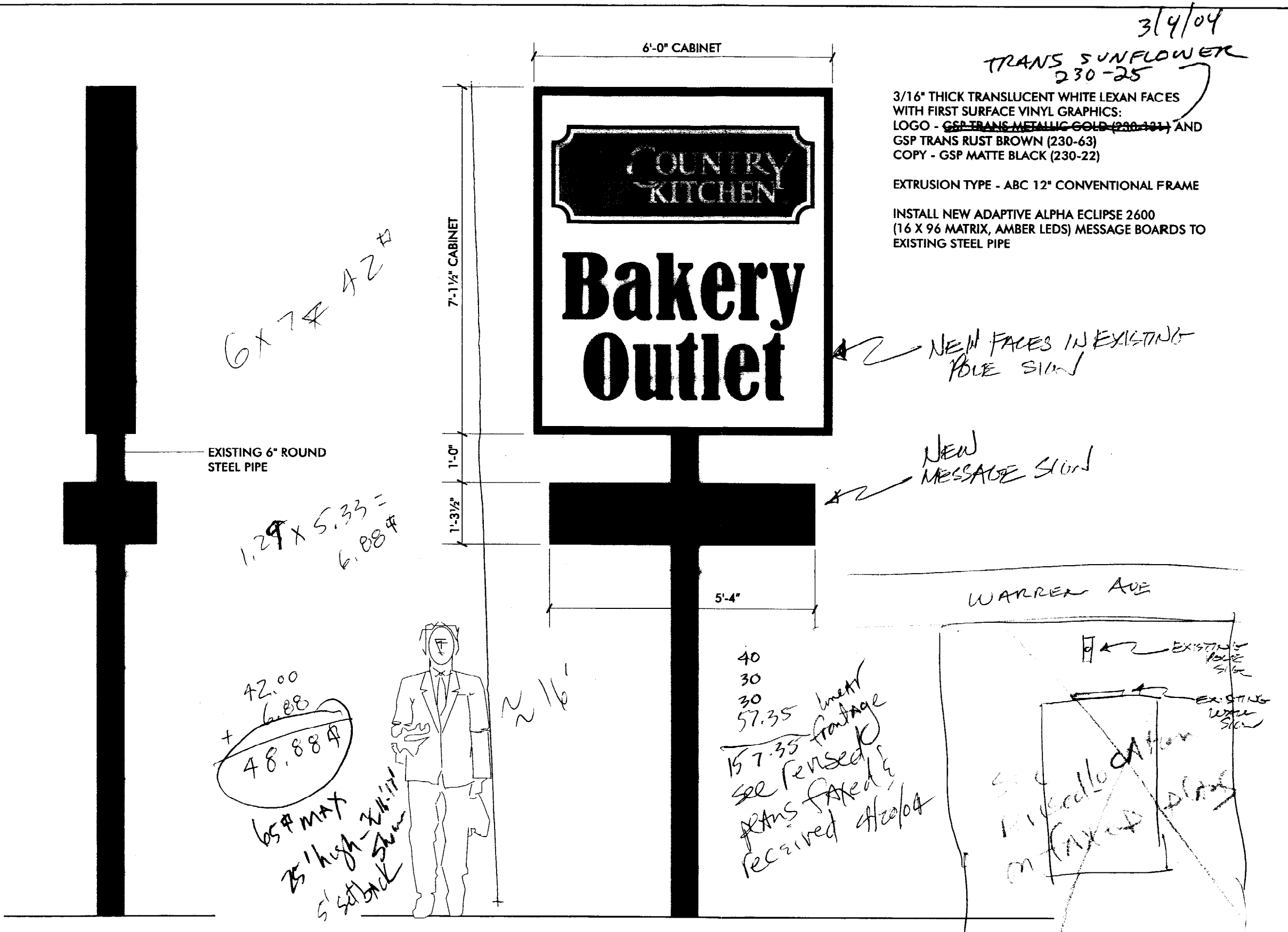
END VIEW SCALE: 1/2" = 1'-0"
