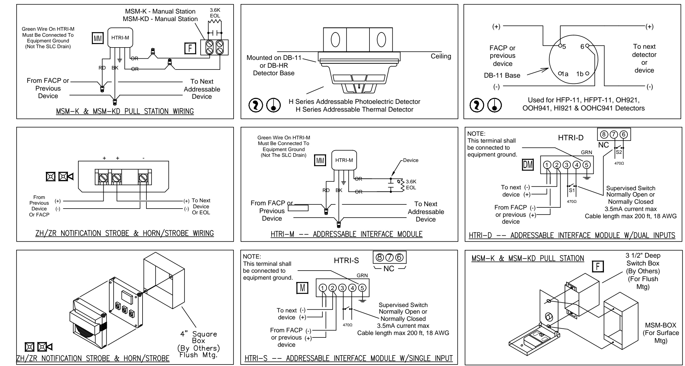
DEVICE WIRING DETAIL SCALE: N.T.S.
