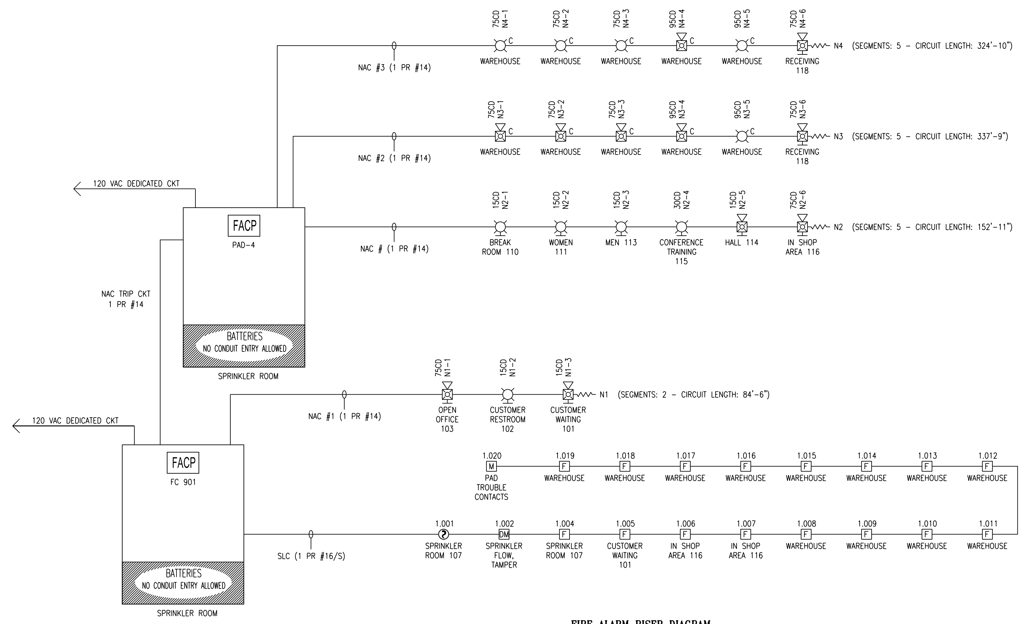
FIRE ALARM RISER DIAGRAM SCALE: N.T.S.
