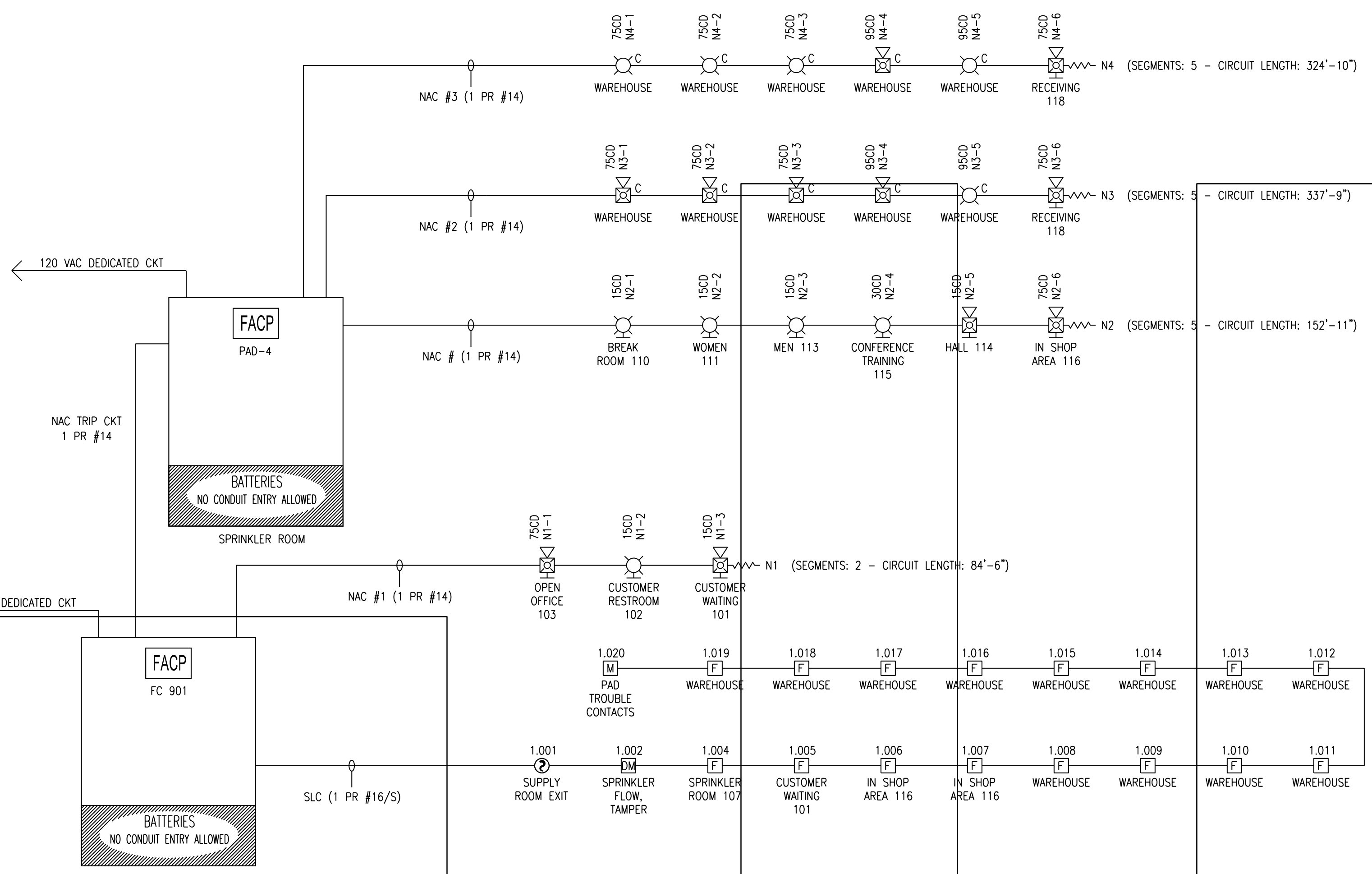
FIRE ALARM RISER DIAGRAM SCALE: N.T.S.
