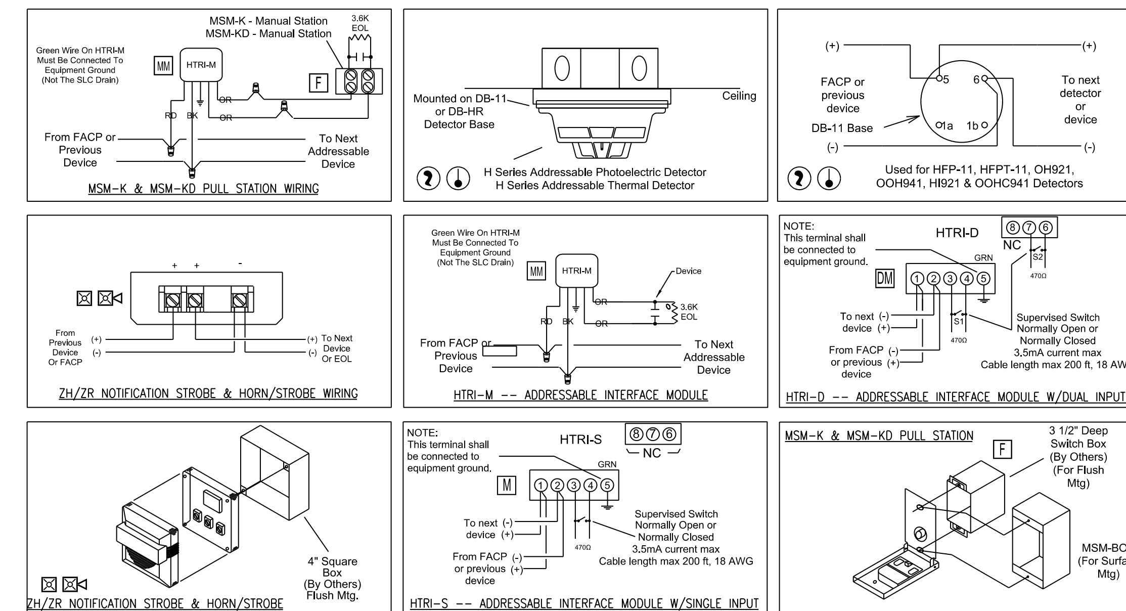
DEVICE WIRING DETAIL SCALE: N.T.S.
