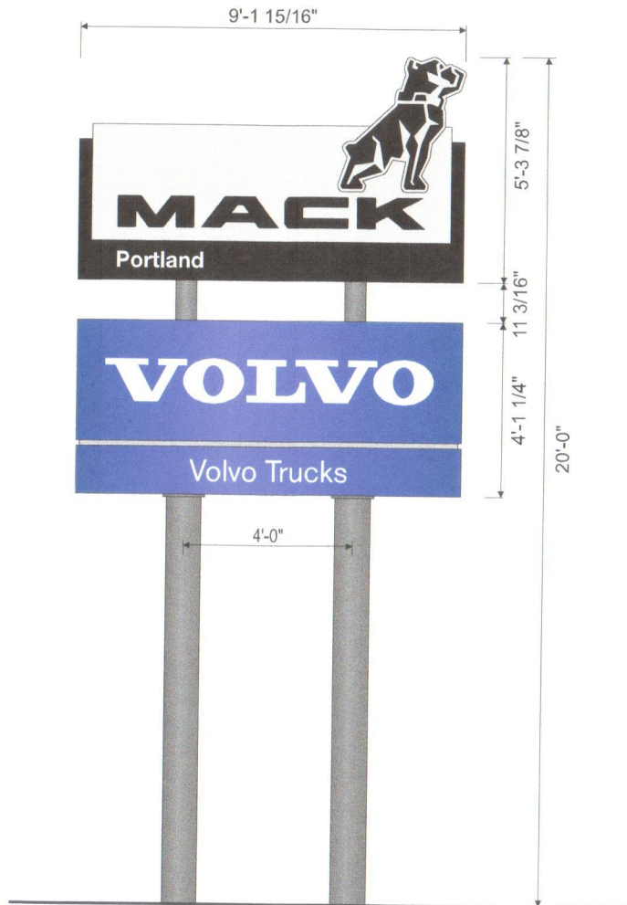
NMP-40(D) / 2800+1 Pylon Sign Scale 1/4" = 1'-0"
