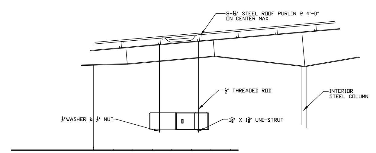
1 FURNACE HANGING DETAIL SCALE: N.T.S.
