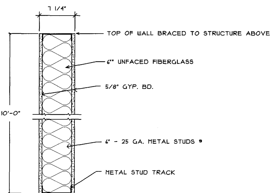
3 BATHROOM WET WALL SCALE: 1" = 1'-0"
