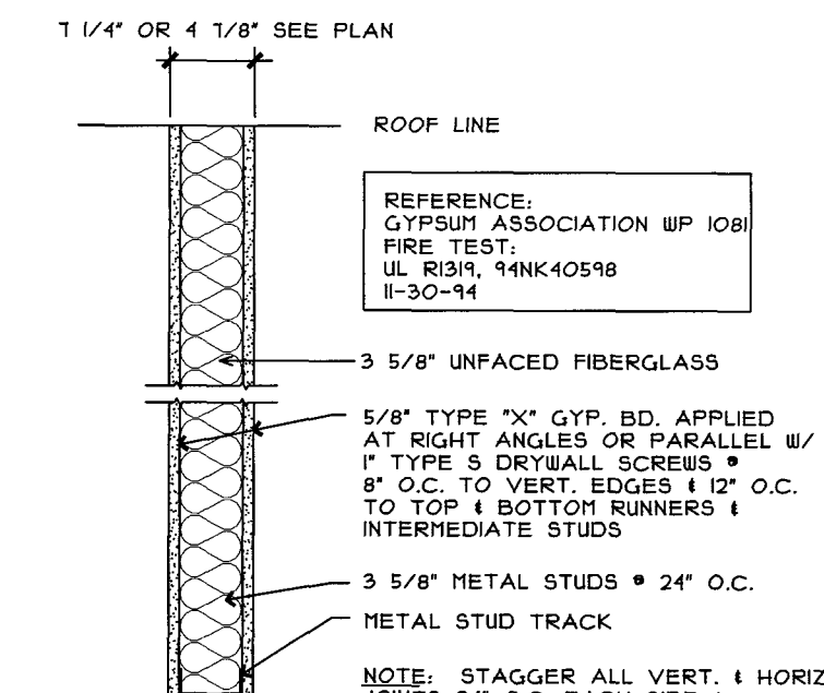
2 1 HR. PARTITION UL DESIGN: U465 SCALE: 1" = 1'-0"
