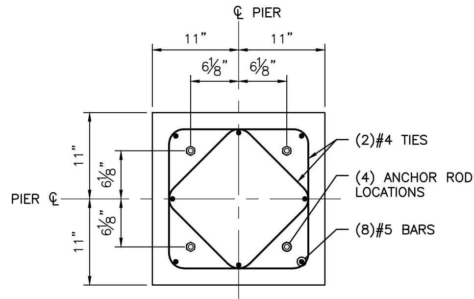
2 PIER DETAIL SK-001 SCALE: 1" = 1'-0"
