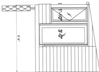
Right Elevation
