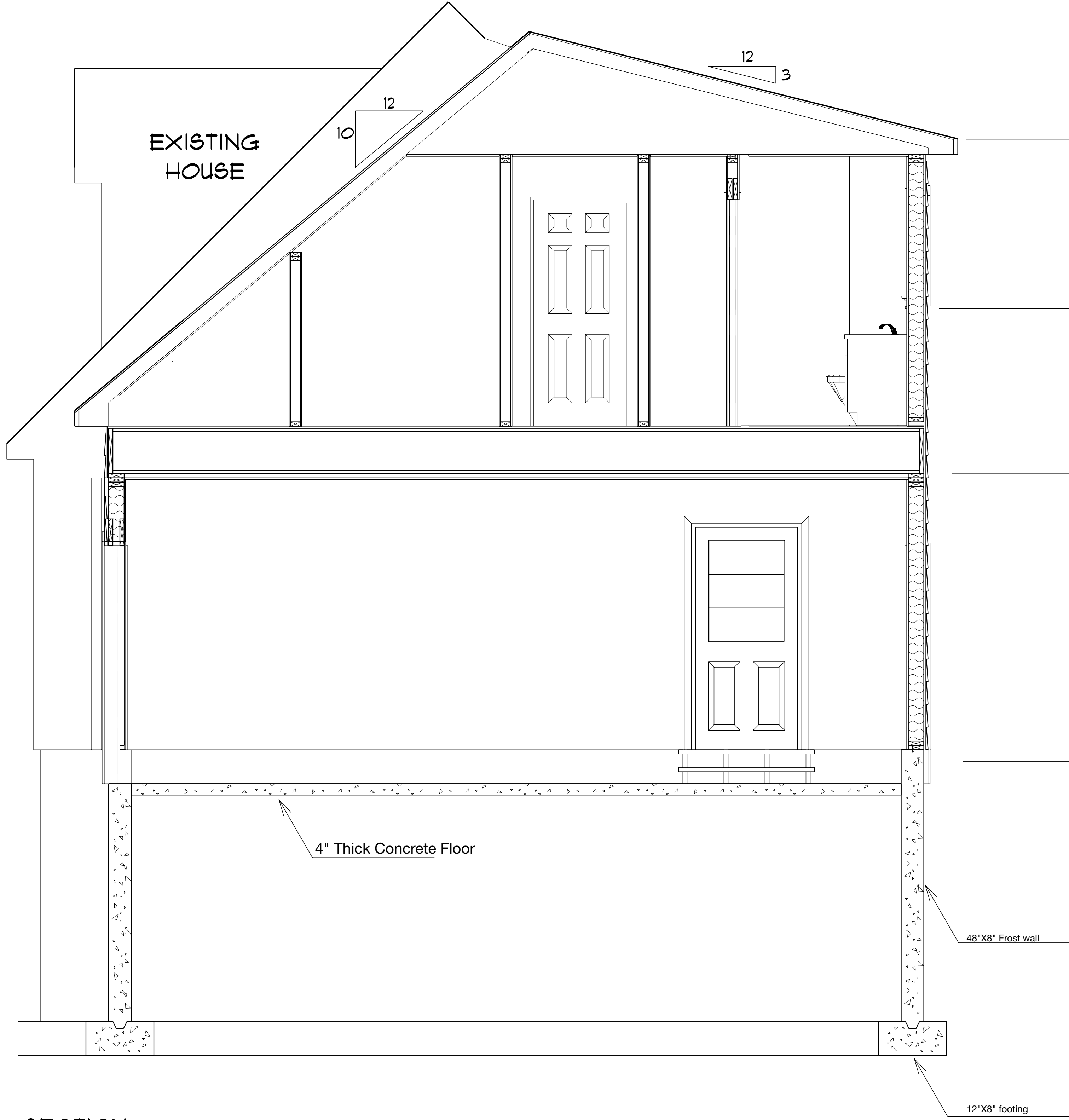
SECTION SCALE: 1/2" = 1'-0"
